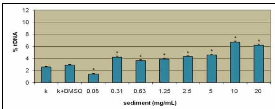
Slika 13. Ošte enje DNA u PLHC-1 stanicama prikazano kao % tDNA ( \bar{x} \pm SD ) u ovisnosti o koncentraciji ekstrakta sedimenta s postaje Ina Rafinerija nafte na Mlaci ekstrahiranog s diklormetanom, k - kontrola, p 0,05 (*).
