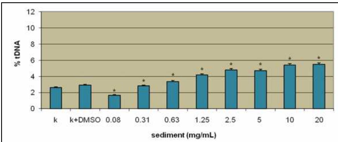
Slika 6. Ošte enje DNA u PLHC-1 stanicama prikazano kao % tDNA ( \bar{x} \pm \text{SEM} ) u ovisnosti o koncentraciji ekstrakta sedimenta s postaje Brodogradilište 3. Maj, k - kontrola, p 0,05 (*).
