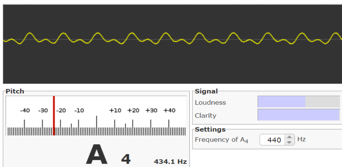
Slika 5.1. Online štimer [14].
