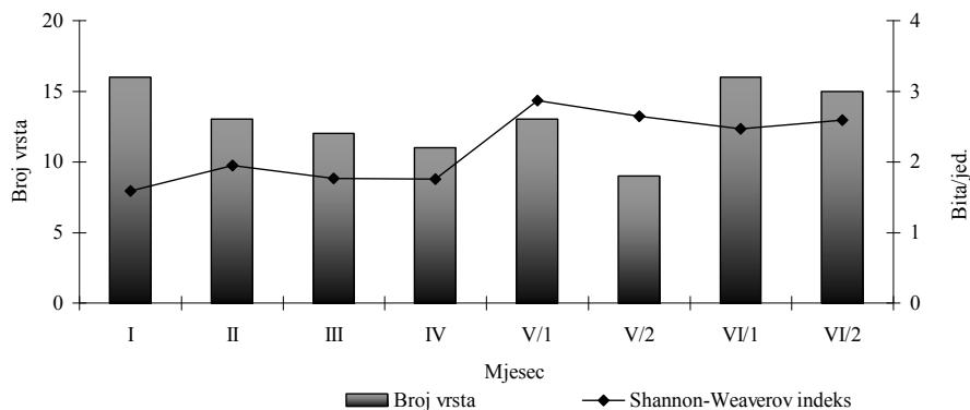
Slika 6 Vremenske promjene Shannon-Weaverovog indeksa raznolikosti ( H' ) na postaji PL
