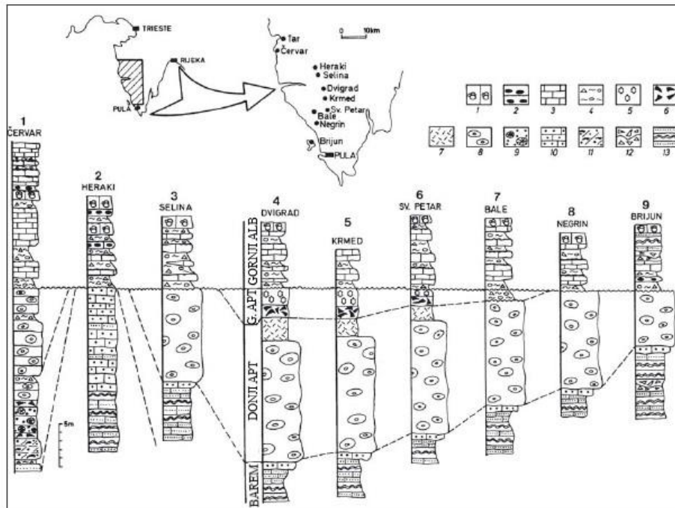
Slika 3.2. Korelacija donjokrednih naslaga (barem–gornji alb) u Istri s različitim trajanjem aptsko/albske emerezije (Velić i dr., 1989; djelomično izmijenjeno).
