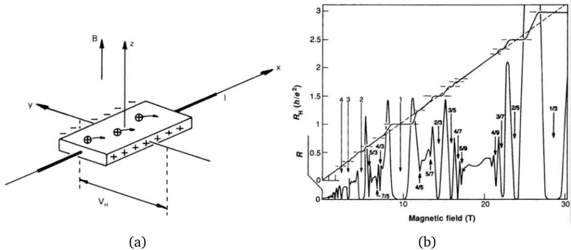
Slika 3.2: a) Princip Hallovog eksperimenta. Struja teče u smjeru x osi, magnetsko polje je u smjeru z osi i javlja se transverzalni napon V_H između točaka različitih y koordinata. b) Kvantni Hallov efekt. Na visokim poljima javljaju se platoi u grafu i Hallov otpor R_H više ne ovisi linearno o B . Na grafu je prikazana i ovisnost longitudinalnog otpora R o polju koji pada na platoima. Strelicama su označeni \nu . Preuzeto sa [9]
