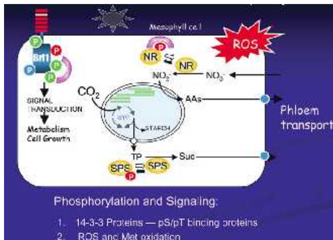
Slika 1. Pojednostavljeni prikaz fosforilacijskih puteva tijekom sinteze aminokiselina i ugljikohidrata u modelu lista sa jednim kloroplastom. NR-nitrat reduktaza; SPS-saharozna fosfat sintaza; Bri1- BRASSINOSTEROID-INSENSITIVE 1
