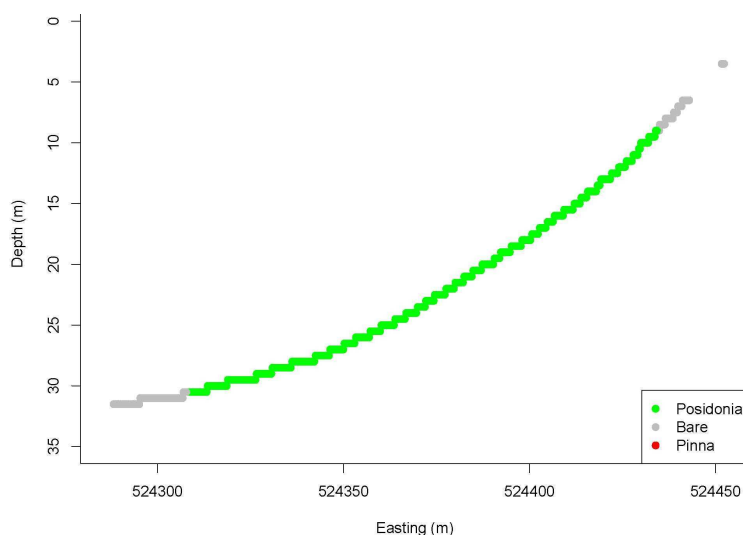
Slika 14. Profil dubine duž video-transekta tr3.5 napravljenog 9. lipnja 2009. godine. Na slici se jasno vidi raspon dubine u kojem je prisutna posidonija (zelena boja): od 9,0 m sve do maksimalne dubine od 30,5 m. Periske nisu uočene.
