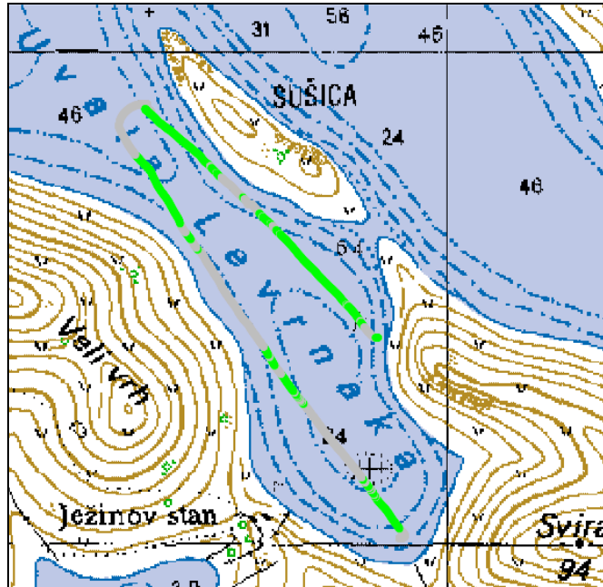
Slika 31. Transekt tr1 snimljen podmorskom geo-referenciranom video-metodom u uvali Levrnaka na otoku Levrnaka 6. prosinca 2009. godine, preklopljen s nautičkom kartom.
