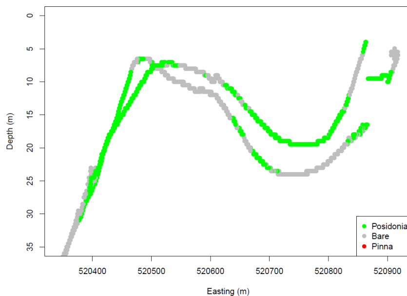
Slika 32. Profil dubine duž video-transekta tr1 napravljenog u uvali Levrnaka u NP Kornati 6. prosinca 2009. godine. Posidonija (zelena boja) se na ovom transektu pojavljuje na maksimalnoj dubini od 31 m i to je najveća dubina na kojoj je posidonija zabilježena u našem istraživanju.
