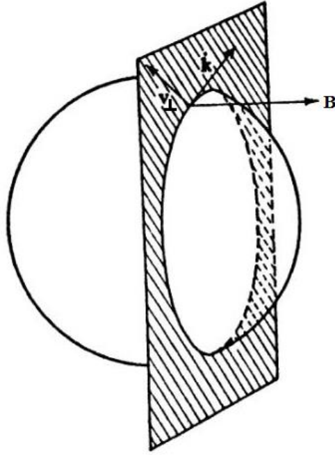
Slika 3.1. Orbita elektrona u magnetskom polju. Fermijeva površina presječena je ravninom okomitom na magnetsko polje, a presječna je kružnica, jedna dozvoljena orbita elektrona. Vektor \vec{k} leži u spomenutoj ravnini i tangencijalan je na orbitu elektrona. Prikazana je promjena elektronskog stanja u vremenu pod utjecajem magnetskog polja. Brzina elektrona \vec{v} okomita je na ekvieni energetsku plohu, a brzina v_{\perp} na orbitu elektrona pri čemu se nalazi u ravnini okomitoj na \vec{B} . [6]
