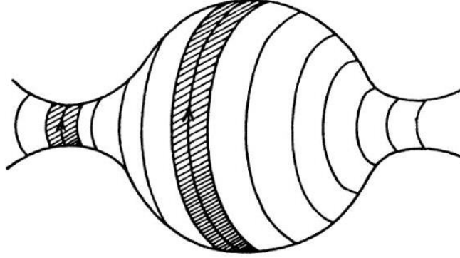
Slika 3.5. Orbite elektrona na dijelovima Fermijeve površine uvijek su u smjeru okomitom na magnetsko polje i prikazane su kružnicama. Ekstremalne orbite Fermijeve površine su najmanjeg ili najvećeg poprečnog presjeka okomito na primijenjeno magnetsko polje i na slici su istaknute šrafiranim područjem oko same orbite. Smjer obilaska elektrona po orbiti naznačen je strelicom. Promjenom smjera magnetskog polja može se odrediti ekstremalne presjeke Fermijeve površine u različitim smjerovima i rekonstruirati oblik Fermijeve površine. [6]
