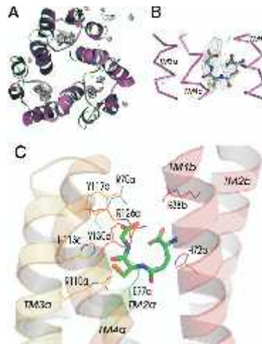
Slika 7. Prikaz vezanja GSH u mPGES-1. A) Pogled odozgo s citoplazmatske strane na mjesta vezanja GSH na trimer mPGES-1. B) GSH u obliku slova U izme u transmembranskih zavojnica 1 i 4 (TM1 i TM4) dviju podjedinica. C) Lanci uklju eni u stvaranje veznog džepa za GSH. Preuzeto iz Jegersshöld i sur., 2008.
