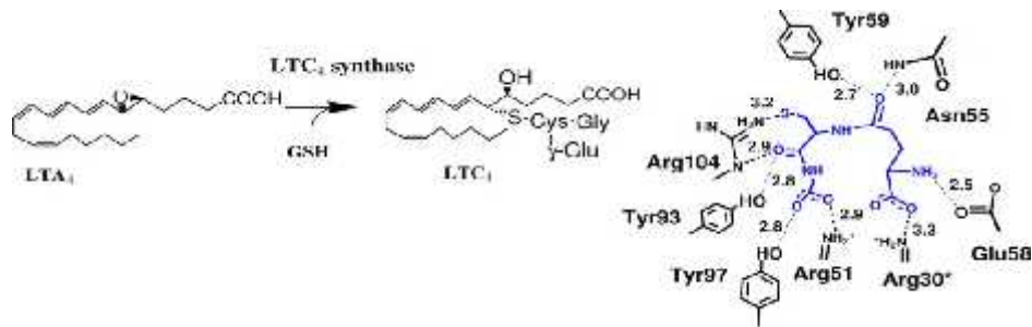
Slika 6. Lijevo, katalitička reakcija LTC 4 sintaze. Desno, aktivacija tiolne skupine GSH pomoću Arg-104. GSH je označen plavom bojom. Preuzeto iz Rinaldo-Matthis i sur., 2010.
