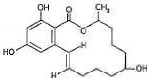
Slika 10. Zearalenon
