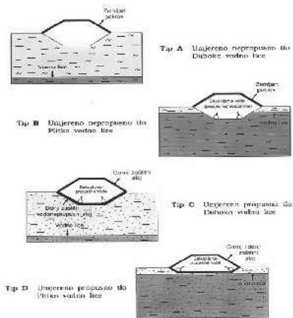
Slika 1. osnovne kombinacije hidrogeoloških osobina i dizajna odlagališta ( http://geol.pmf.hr/~mjuracic/predavanja/Geol.zastite.okolisa/07.Odlagalista.otpada.pdf , Lisk 1991.)
