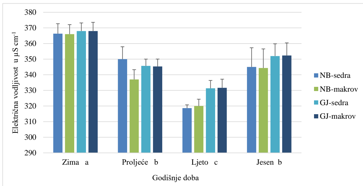
Slika 23. Srednje vrijednosti električne vodljivosti ( \pm SD) na mikrolokacijama po godišnjim dobima. Različita slova uz godišnja doba označavaju statistički značajnu razliku kod p<0,001 prema post-hoc Tukey HSD testu
