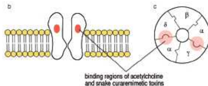
Slika 5. Longitudinalni i transverzalni presjek nikotinskog acetilkolinskog receptora u membrani
