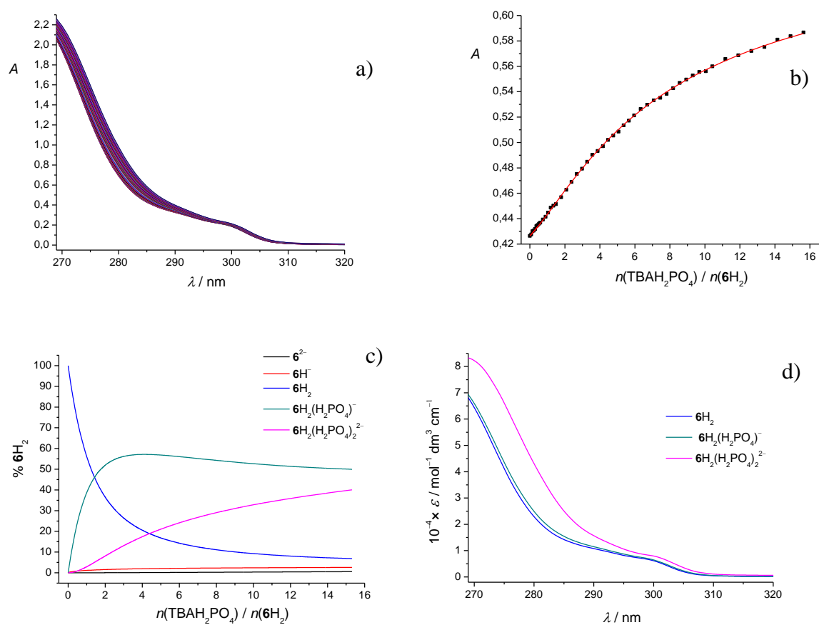
Slika 64. a) Spektrofotometrijska titracija 6H_2 ( c = 3,01 \times 10^{-5} mol dm ^{-3} ) s TBAH_2PO_4 ( c = 1,04 \times 10^{-3} mol dm ^{-3} ) u DMSO. Spektri su korigirani za razrjeđenje. l = 1 cm, (25,0 \pm 0,1) °C. b) Ovisnost apsorbancije otopine 6H_2 pri 285 nm o množinskom omjeru n(TBAH_2PO_4) / n(6H_2) . ■ izmjerene vrijednosti, — izračunane vrijednosti. c) Distribucija pojedinih vrsta tijekom titracije otopine 6H_2 s TBAH_2PO_4 . d) Karakteristični UV spektri spoja 6H_2 i njegovih kompleksa s dihidrogenfosfatom.
