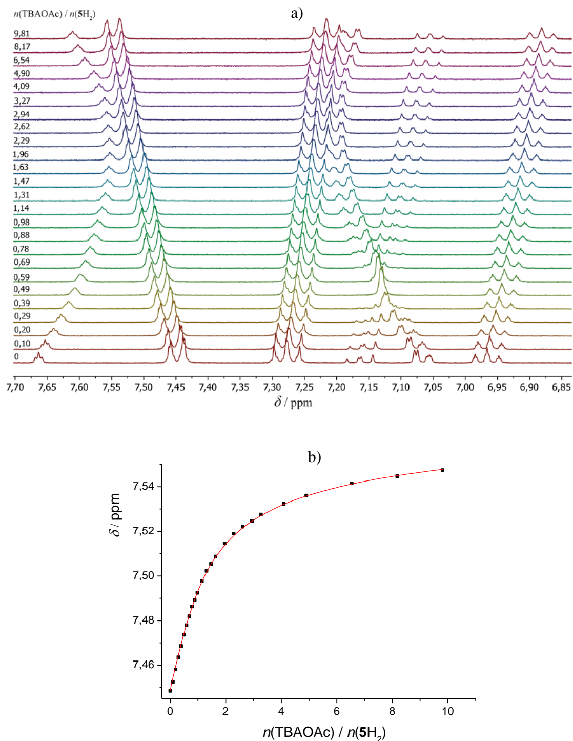
Slika 59. a) ^1\text{H} NMR titracija 5\text{H}_2 ( c = 6,00 \times 10^{-4} \text{ mol dm}^{-3} ) s TBAOAc ( c = 1,03 \times 10^{-2} \text{ mol dm}^{-3} ) u \text{DMSO-}d_6 pri (25,0 \pm 0,1) \text{ }^\circ\text{C} . b) Ovisnost kemijskog pomaka \text{H}_a protona tijekom ^1\text{H} NMR titracije s TBAOAc o množinskom omjeru n(\text{TBAOAc}) / n(5\text{H}_2) . ■ izmjerene vrijednosti, — izračunane vrijednosti.
