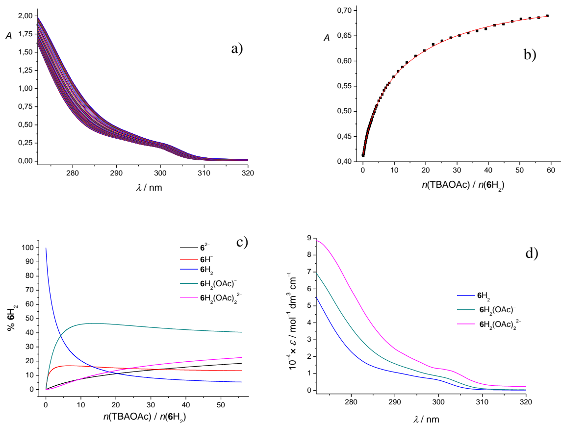
Slika 56. a) Spektrofotometrijska titracija 6\text{H}_2 ( c = 2,92 \times 10^{-5} \text{ mol dm}^{-3} ) s TBAOAc ( c = 3,79 \times 10^{-3} \text{ mol dm}^{-3} ) u DMSO. Spektri su korigirani za razrjeđenje. l = 1 \text{ cm} , \check{Z}(25,0 \pm 0,1) \text{ }^\circ\text{C} . b) Ovisnost apsorbancije otopine 6\text{H}_2 pri 285 nm o množinskom omjeru n(\text{TBAOAc}) / n(6\text{H}_2) . ■ izmjerene vrijednosti, — izračunane vrijednosti. c) Distribucija pojedinih vrsta tijekom titracije otopine 6\text{H}_2 s TBAOAc. d) Karakteristični UV spektri spoja 6\text{H}_2 i njegovih kompleksa s acetatom.
