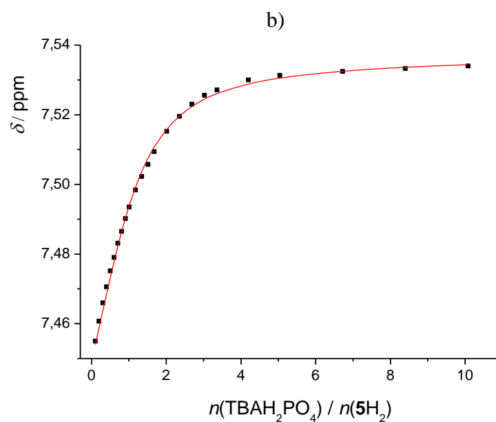
Slika 69. a) ^1\text{H} NMR titracija \text{5H}_2 ( c = 6,00 \times 10^{-4} \text{ mol dm}^{-3} ) s \text{TBAH}_2\text{PO}_4 ( c = 1,02 \times 10^{-2} \text{ mol dm}^{-3} ) u \text{DMSO-}d_6 pri (25,0 \pm 0,1) \text{ }^\circ\text{C} . b) Ovisnost kemijskog pomaka \text{H}_d protona tijekom ^1\text{H} NMR titracije s \text{TBAH}_2\text{PO}_4 o množinskom omjeru n(\text{TBAH}_2\text{PO}_4) / n(\text{5H}_2) . ■ izmjerene vrijednosti, — izračunane vrijednosti.
