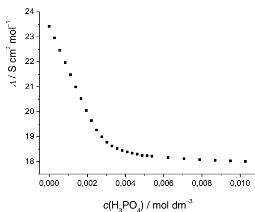
Slika 20. Konduktometrijska titracija otopine TBAH 2 PO 4 ( c = 3,0 \times 10^{-2} \text{ mol dm}^{-3} ) s H 3 PO 4 ( c = 0,113 \text{ mol dm}^{-3} ) u DMSO pri (25,0 \pm 0,1) ^\circ\text{C} .
