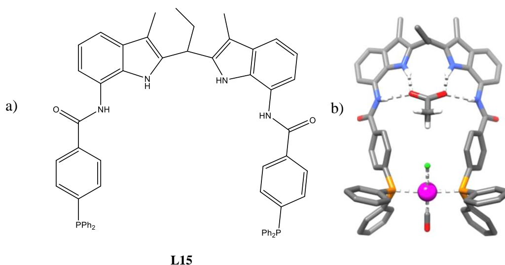
Slika 12. a) Struktura receptora L15 i b) struktura rodijevog supramolekulskog kompleksa [\text{Rh}(\text{L15}\cdot\text{OAc})(\text{CO})\text{Cl}]^- koji sudjeluje u katalitičkoj reakciji hidroformilacije nezasićenih karboksilnih kiselina. 32b
