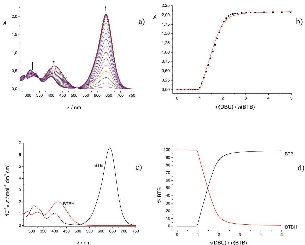
Slika 27. a) Spektrofotometrijska titracija brotmol plavog ( c = 3,19 \times 10^{-5} \text{ mol dm}^{-3} ) s DBU ( c = 2,37 \times 10^{-3} \text{ mol dm}^{-3} ) u DMSO. Spektri su korigirani za razrjeđenje. l = 1 \text{ cm} , (25,0 \pm 0,1) \text{ }^\circ\text{C} . b) Ovisnost apsorbancije otopine brotmol plavog pri 638 nm o množinskom omjeru n(\text{DBU}) / n(\text{BTB}) . ■ izmjerene vrijednosti, — izračunane vrijednosti. c) Karakteristični UV-Vis spektri protonirane i deprotonirane forme brotmol plavog. d) Distribucija pojedinih vrsta tijekom titracije otopine brotmol plavog s DBU.
