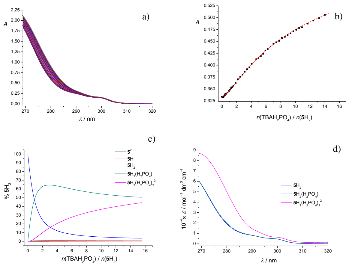
Slika 63. a) Spektrofotometrijska titracija 5\text{H}_2 ( c = 3,05 \times 10^{-5} \text{ mol dm}^{-3} ) s \text{TBAH}_2\text{PO}_4 ( c = 1,10 \times 10^{-3} \text{ mol dm}^{-3} ) u DMSO. Spektri su korigirani za razrjeđenje. l = 1 \text{ cm} , (25,0 \pm 0,1) \text{ }^\circ\text{C} . b) Ovisnost apsorbancije otopine 5\text{H}_2 pri 285 nm o množinskom omjeru n(\text{TBAH}_2\text{PO}_4) / n(5\text{H}_2) . ■ izmjerene vrijednosti, — izračunane vrijednosti. c) Distribucija pojedinih vrsta tijekom titracije otopine 5\text{H}_2 s \text{TBAH}_2\text{PO}_4 . d) Karakteristični UV spektri spoja 5\text{H}_2 i njegovih kompleksa s dihidrogenfosfatom.
