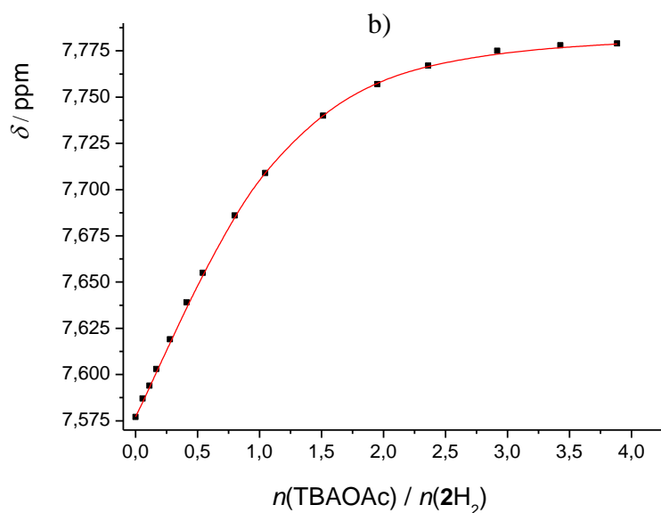
Slika 41. a) ^1\text{H} NMR titracija 2\text{H}_2 ( c = 6,10 \times 10^{-4} \text{ mol dm}^{-3} ) s TBAOAc ( c = 8,61 \times 10^{-3} \text{ mol dm}^{-3} ) u \text{DMSO-}d_6 pri (25,0 \pm 0,1) \text{ }^\circ\text{C} . b) Ovisnost kemijskog pomaka \text{H}_b protona tijekom ^1\text{H} NMR titracije s TBAOAc o množinskom omjeru n(\text{TBAOAc}) / n(2\text{H}_2) . ■ izmjerene vrijednosti, — izračunane vrijednosti.
