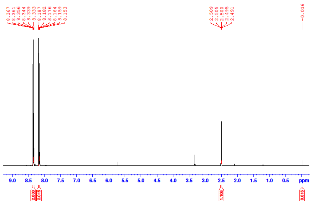
Slika P30. 1 H NMR spektar spoja P1 u DMSO- d 6 (400 MHz).
