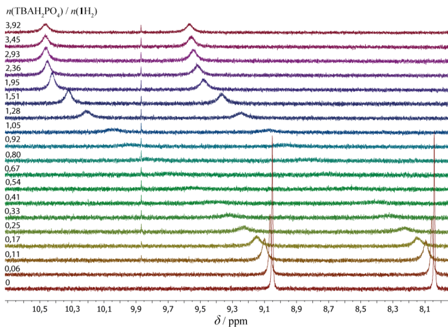
Slika P59. Kemijski pomaci protona ureidne skupine tijekom ^1\text{H} NMR titracije 1\text{H}_2 ( c = 5,95 \times 10^{-4} \text{ mol dm}^{-3} ) s TBAH _2 PO _4 ( c = 8,78 \times 10^{-3} \text{ mol dm}^{-3} ) u DMSO- d_6 pri (25,0 \pm 0,1) ^\circ\text{C} .
