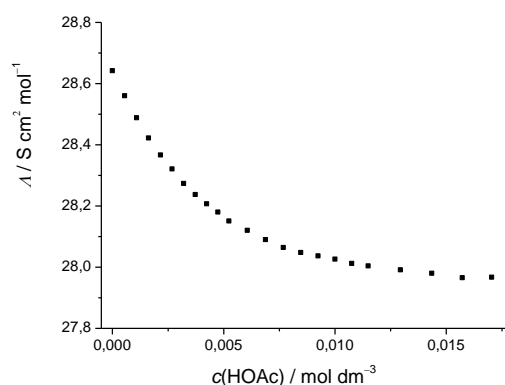
Slika 19. Konduktometrijska titracija otopina TBAOAc ( c = 3,0 \times 10^{-2} \text{ mol dm}^{-3} ) s HOAc ( c = 0,11 \text{ mol dm}^{-3} ) u DMSO pri (25,0 \pm 0,1) ^\circ\text{C} .
