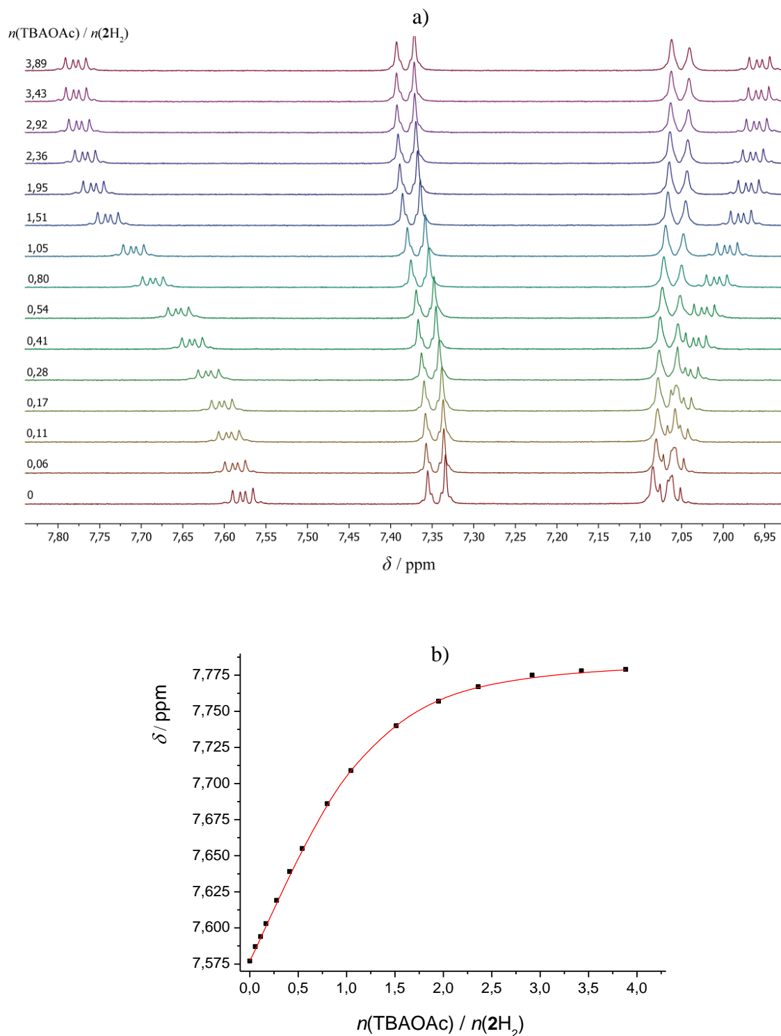
Slika 41. a) ^1\text{H} NMR titracija 2\text{H}_2 ( c = 6,10 \times 10^{-4} \text{ mol dm}^{-3} ) s TBAOAc ( c = 8,61 \times 10^{-3} \text{ mol dm}^{-3} ) u \text{DMSO-}d_6 pri (25,0 \pm 0,1) \text{ }^\circ\text{C} . b) Ovisnost kemijskog pomaka \text{H}_b protona tijekom ^1\text{H} NMR titracije s TBAOAc o množinskom omjeru n(\text{TBAOAc}) / n(2\text{H}_2) . ■ izmjerene vrijednosti, — izračunane vrijednosti.
