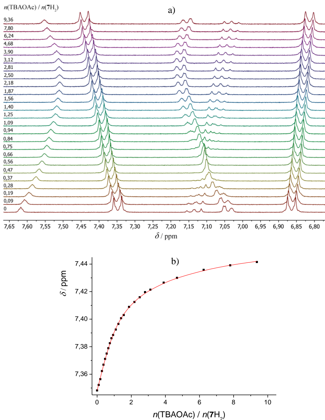
Slika 61. a) ^1\text{H} NMR titracija 7\text{H}_2 ( c = 6,29 \times 10^{-4} \text{ mol dm}^{-3} ) s TBAOAc ( c = 1,03 \times 10^{-2} \text{ mol dm}^{-3} ) u \text{DMSO-}d_6 pri (25,0 \pm 0,1) \text{ }^\circ\text{C} . b) Ovisnost kemijskog pomaka \text{H}_a protona tijekom ^1\text{H} NMR titracije s TBAOAc o množinskom omjeru n(\text{TBAOAc}) / n(7\text{H}_2) . ■ izmjerene vrijednosti, — izračunane vrijednosti.
