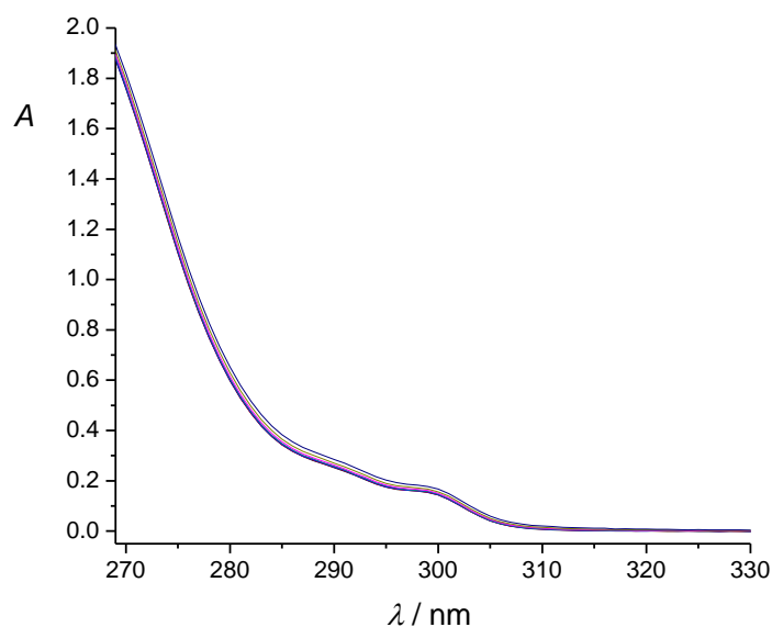
Slika P40. Spektrofotometrijska titracija 5\text{H}_2 ( c = 3,05 \times 10^{-5} \text{ mol dm}^{-3} ) s otopinom \text{TEACl} ( c = 6,89 \times 10^{-3} \text{ mol dm}^{-3} ) u DMSO. Spektri su korigirani za razrjeđenje. Množinski omjer n(\text{TEACl}) / n(5\text{H}_2) na kraju titracije iznosi 98. l = 1 \text{ cm} , (25,0 \pm 0,1) \text{ }^\circ\text{C} .
