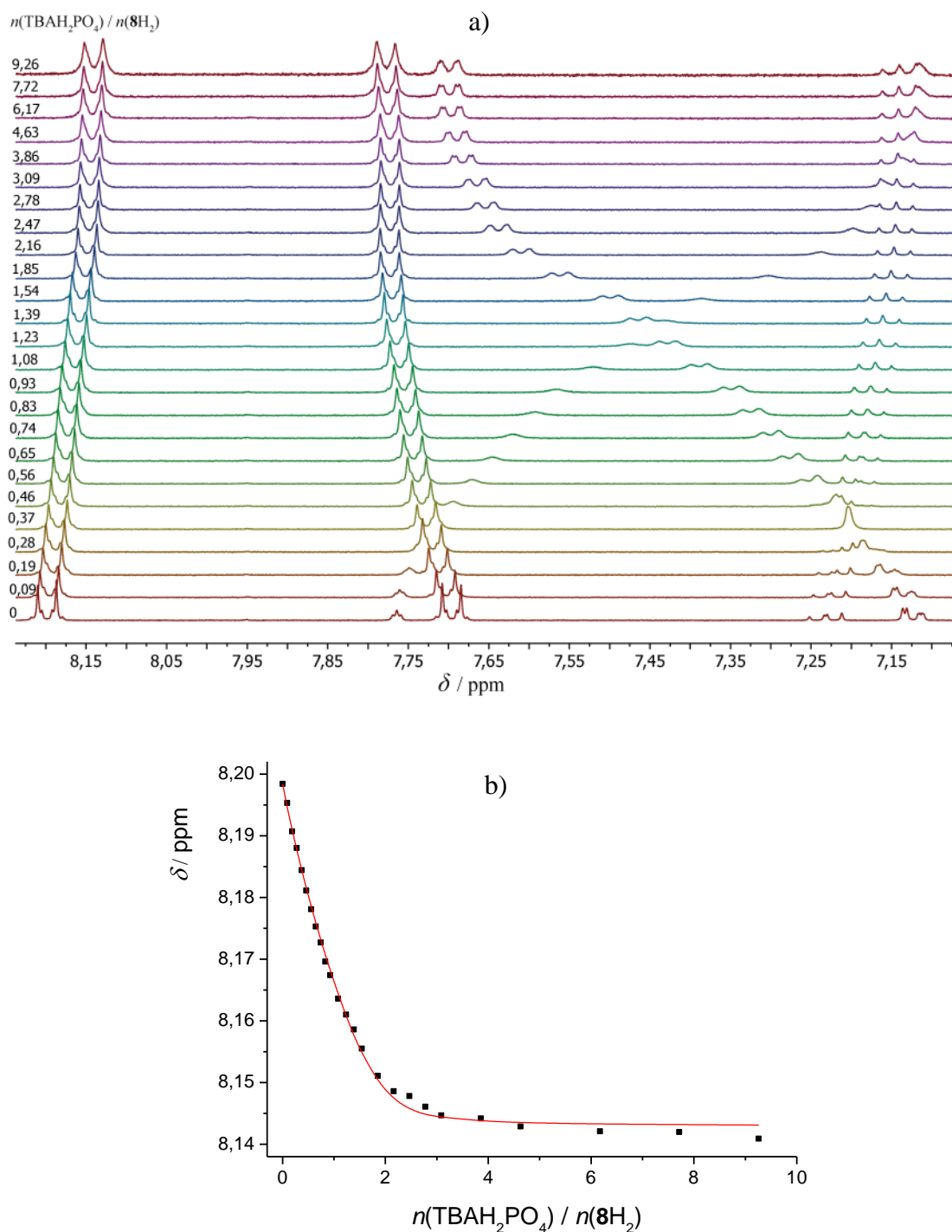
Slika 72. a) ^1\text{H} NMR titracija \mathbf{8H}_2 ( c = 5,86 \times 10^{-4} \text{ mol dm}^{-3} ) s \text{TBAH}_2\text{PO}_4 ( c = 9,49 \times 10^{-3} \text{ mol dm}^{-3} ) u \text{DMSO-}d_6 pri (25,0 \pm 0,1) ^\circ\text{C} . b) Ovisnost kemijskog pomaka \text{H}_c protona tijekom ^1\text{H} NMR titracije s \text{TBAH}_2\text{PO}_4 o množinskom omjeru n(\text{TBAH}_2\text{PO}_4) / n(\mathbf{8H}_2) . ■ izmjerene vrijednosti, — izračunane vrijednosti.
