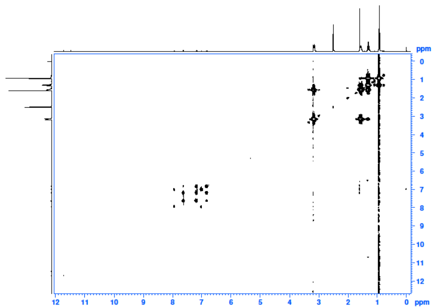
Slika P73. COSY spektar spoja 5H_2 s TBAOAc u DMSO-d_6 ( n(TBAOAc) / n(5H_2) \approx 15 ) (400 MHz).
