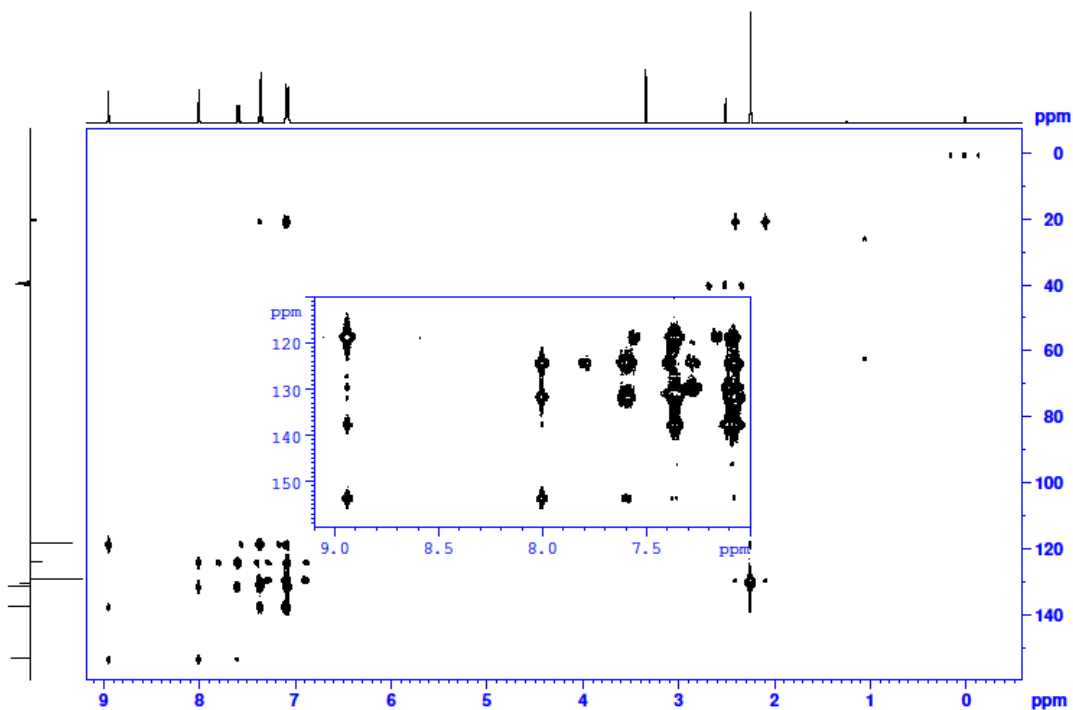
Slika P7. HMBC spektar spoja 2H_2 u DMSO- d_6 (400 MHz).
