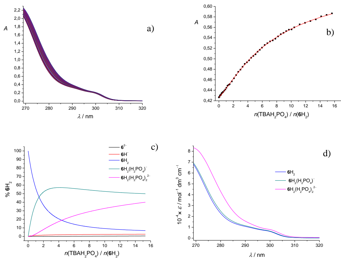
Slika 64. a) Spektrofotometrijska titracija 6H_2 ( c = 3,01 \times 10^{-5} \text{ mol dm}^{-3} ) s TBAH_2PO_4 ( c = 1,04 \times 10^{-3} \text{ mol dm}^{-3} ) u DMSO. Spektri su korigirani za razrjeđenje. l = 1 \text{ cm} , (25,0 \pm 0,1) \text{ }^\circ\text{C} . b) Ovisnost apsorbancije otopine 6H_2 pri 285 nm o množinskom omjeru n(TBAH_2PO_4) / n(6H_2) . ■ izmjerene vrijednosti, — izračunane vrijednosti. c) Distribucija pojedinih vrsta tijekom titracije otopine 6H_2 s TBAH_2PO_4 . d) Karakteristični UV spektri spoja 6H_2 i njegovih kompleksa s dihidrogenfosfatom.
