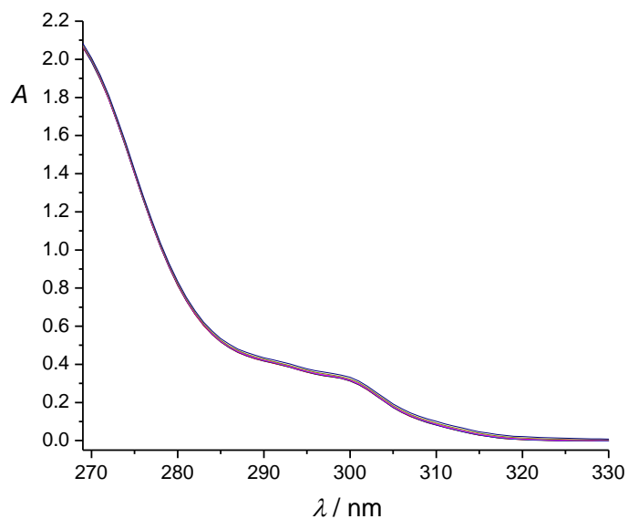
Slika P48. Spektrofotometrijska titracija 7H_2 ( c = 3,03 \times 10^{-5} \text{ mol dm}^{-3} ) s otopinom TBANO_3 ( c = 7,01 \times 10^{-3} \text{ mol dm}^{-3} ) u DMSO. Spektri su korigirani za razrjeđenje. Množinski omjer n(TBANO_3) / n(7H_2) na kraju titracije iznosi 100. l = 1 \text{ cm} , (25,0 \pm 0,1) \text{ }^\circ\text{C} .
