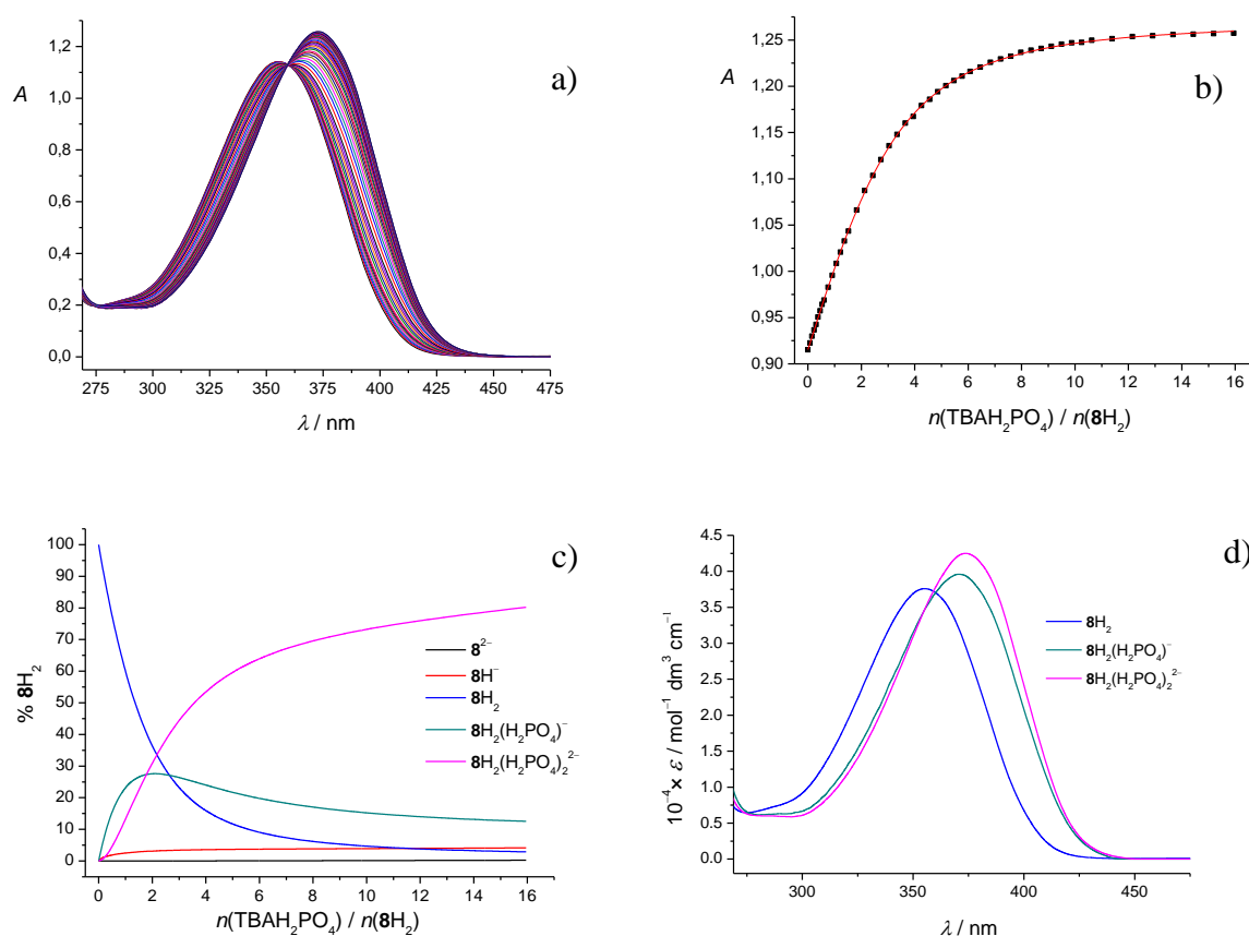
Slika 66. a) Spektrofotometrijska titracija 8H_2 ( c = 3,04 \times 10^{-5} \text{ mol dm}^{-3} ) s TBAH_2PO_4 ( c = 1,07 \times 10^{-3} \text{ mol dm}^{-3} ) u DMSO. Spektri su korigirani za razrjeđenje. l = 1 \text{ cm} , (25,0 \pm 0,1) \text{ }^\circ\text{C} . b) Ovisnost apsorbancije otopine 8H_2 pri 373 nm o množinskom omjeru n(TBAH_2PO_4) / n(8H_2) . ■ izmjerene vrijednosti, — izračunane vrijednosti. c) Distribucija pojedinih vrsta tijekom titracije otopine 8H_2 s TBAH_2PO_4 . d) Karakteristični UV-Vis spektri spoja 8H_2 i njegovih kompleksa s dihidrogenfosfatom.
