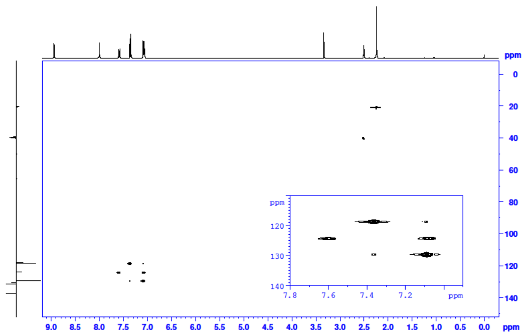
Slika P6. HSQC spektar spoja 2H_2 u DMSO- d_6 (400 MHz).
