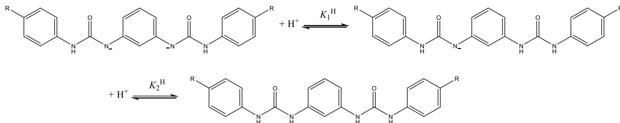
Shema 8. Protonacijske ravnoteže istraživanih ureidnih receptora; L_m = 5, 6, 7 i 8 ; R = H, CH_3, OCH_3 ili NO_2 .
