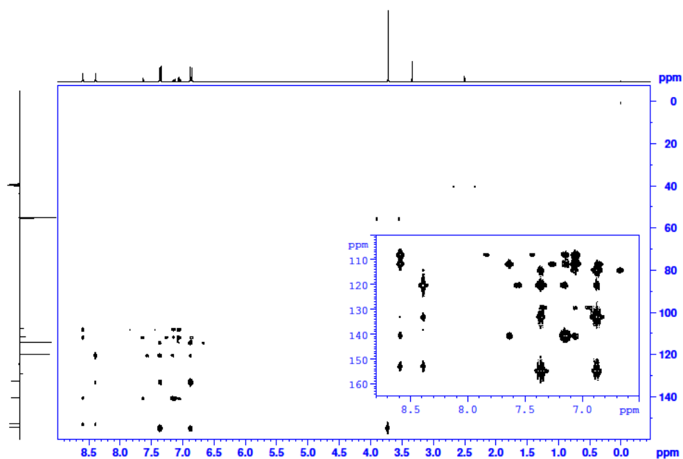
Slika P26. HMBC spektar spoja 7H_2 u DMSO- d_6 (400 MHz).
