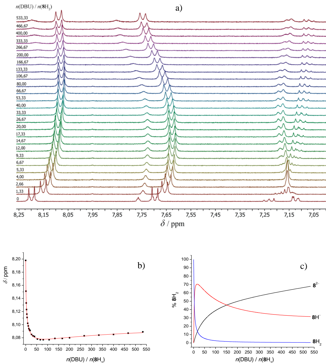
Slika 54. a) ^1H NMR titracija 8H_2 ( c = 5,86 \times 10^{-4} \text{ mol dm}^{-3} ) s DBU ( c = 4,10 \times 10^{-1} \text{ mol dm}^{-3} ) u DMSO- d_6 pri (25,0 \pm 0,1) ^\circ\text{C} . b) Ovisnost kemijskog pomaka H_e protona spoja 8H_2 tijekom ^1H NMR titracije s DBU o množinskom omjeru n(\text{DBU}) / n(8H_2) . ■ izmjerene vrijednosti, — izračunane vrijednosti. c) Distribucija protonacijskih vrsta tijekom titracije otopine 8H_2 s DBU.
