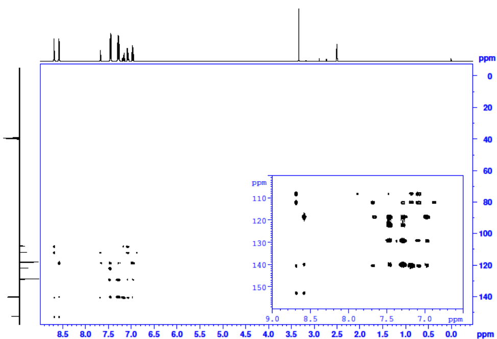
Slika P16. HMBC spektar spoja 5H_2 u DMSO- d_6 (400 MHz).
