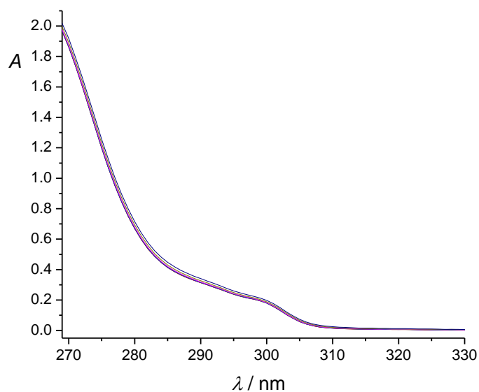
Slika P43. Spektrofotometrijska titracija 6\text{H}_2 ( c = 2,94 \times 10^{-5} \text{ mol dm}^{-3} ) s otopinom TEACl ( c = 6,89 \times 10^{-3} \text{ mol dm}^{-3} ) u DMSO. Spektri su korigirani za razrjeđenje. Množinski omjer n(\text{TEACl}) / n(6\text{H}_2) na kraju titracije iznosi 101. l = 1 \text{ cm} , (25,0 \pm 0,1) \text{ }^\circ\text{C} .
