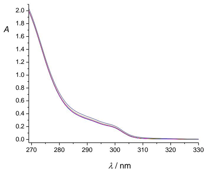
Slika P44. Spektrofotometrijska titracija 6\text{H}_2 ( c = 2,94 \times 10^{-5} \text{ mol dm}^{-3} ) s otopinom TBAClO 4 ( c = 7,04 \times 10^{-3} \text{ mol dm}^{-3} ) u DMSO. Spektri su korigirani za razrjeđenje. Množinski omjer n(\text{TBAClO}_4) / n(6\text{H}_2) na kraju titracije iznosi 103. l = 1 \text{ cm} , (25,0 \pm 0,1) \text{ }^\circ\text{C} .
