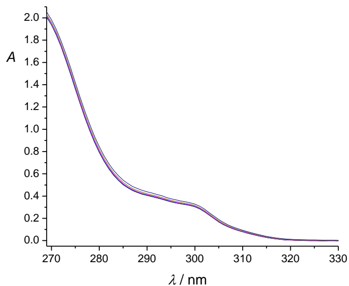
Slika P46. Spektrofotometrijska titracija 7H 2 ( c = 3,03 \times 10^{-5} \text{ mol dm}^{-3} ) s otopinom TEACl ( c = 6,89 \times 10^{-3} \text{ mol dm}^{-3} ) u DMSO. Spektri su korigirani za razrjeđenje. Množinski omjer n(\text{TEACl}) / n(\mathbf{7H}_2) na kraju titracije iznosi 98. l = 1 \text{ cm} , (25,0 \pm 0,1) \text{ }^\circ\text{C} .
