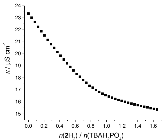
Slika P54. Ovisnost provodnosti otopine TBAH_2PO_4 o množinskom omjeru n(2H_2) / n(TBAH_2PO_4) tijekom konduktometrijske titracije TBAH_2PO_4 ( c = 1,01 \times 10^{-3} \text{ mol dm}^{-3} ) s 2H_2 ( c = 9,99 \times 10^{-3} \text{ mol dm}^{-3} ) u DMSO pri (25,0 \pm 0,1) ^\circ C .
