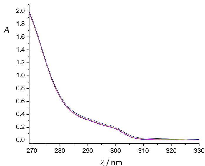
Slika P45. Spektrofotometrijska titracija 6H 2 ( c = 2,94 \times 10^{-5} \text{ mol dm}^{-3} ) s otopinom TBANO 3 ( c = 7,01 \times 10^{-3} \text{ mol dm}^{-3} ) u DMSO. Spektri su korigirani za razrjeđenje. Množinski omjer n(\text{TBANO}_3) / n(\mathbf{6H}_2) na kraju titracije iznosi 103. l = 1 \text{ cm} , (25,0 \pm 0,1) \text{ }^\circ\text{C} .
