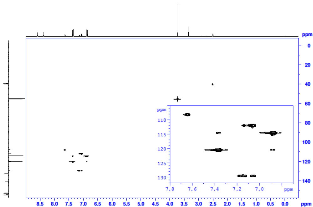
Slika P25. HSQC spektar spoja 7H_2 u DMSO- d_6 (400 MHz).
