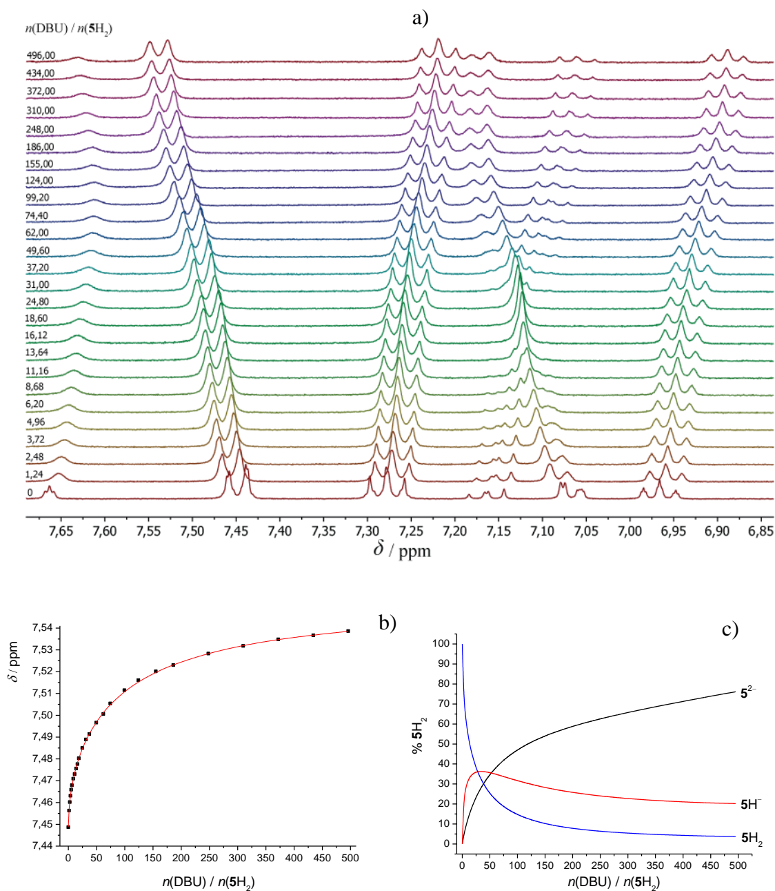
Slika 51. a) ^1H NMR titracija 5H_2 ( c = 6,00 \times 10^{-4} \text{ mol dm}^{-3} ) s DBU ( c = 3,91 \times 10^{-1} \text{ mol dm}^{-3} ) u \text{DMSO-}d_6 pri (25,0 \pm 0,1) \text{ }^\circ\text{C} . b) Ovisnost kemijskog pomaka H_d protona spoja 5H_2 tijekom ^1H NMR titracije s DBU o množinskom omjeru n(\text{DBU}) / n(5H_2) . ■ izmjerene vrijednosti, — izračunane vrijednosti. c) Distribucija protonacijskih vrsta tijekom titracije otopine 5H_2 s DBU.
