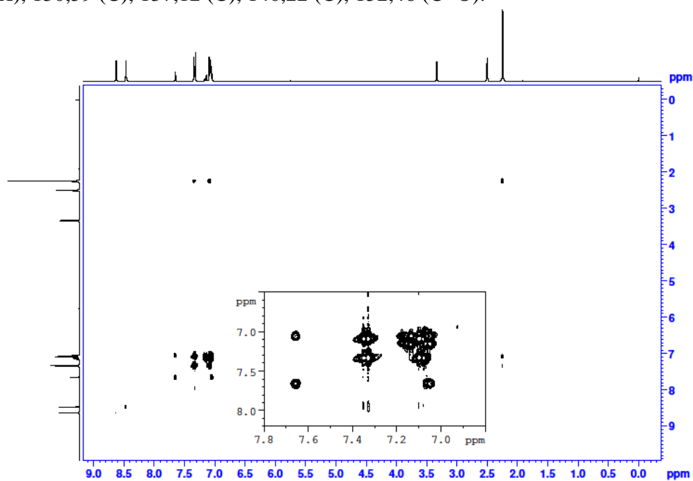
Slika P19. COSY spektar spoja 6\text{H}_2 u \text{DMSO-}d_6 (400 MHz).
