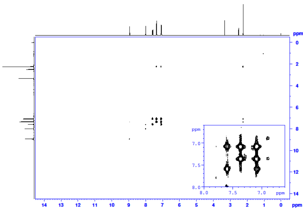
Slika P5. COSY spektar spoja 2\text{H}_2 u \text{DMSO-}d_6 (400 MHz).
