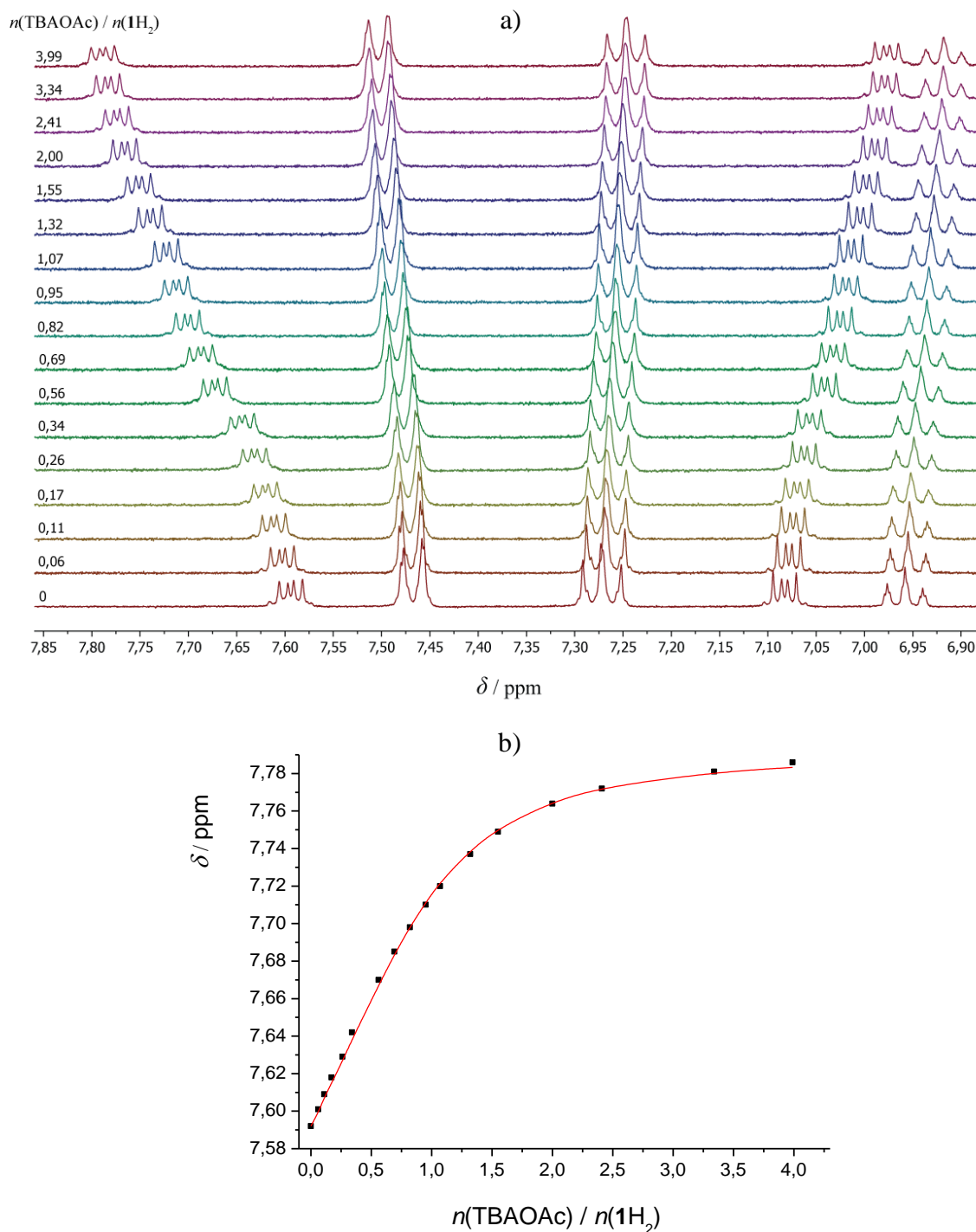
Slika 40. a) ^1\text{H} NMR titracija 1\text{H}_2 ( c = 5,95 \times 10^{-4} \text{ mol dm}^{-3} ) s TBAOAc ( c = 8,61 \times 10^{-3} \text{ mol dm}^{-3} ) u \text{DMSO-}d_6 pri (25,0 \pm 0,1) \text{ }^\circ\text{C} . b) Ovisnost kemijskog pomaka \text{H}_b protona tijekom ^1\text{H} NMR titracije s TBAOAc o množinskom omjeru n(\text{TBAOAc}) / n(1\text{H}_2) . ■ izmjerene vrijednosti, — izračunane vrijednosti.
