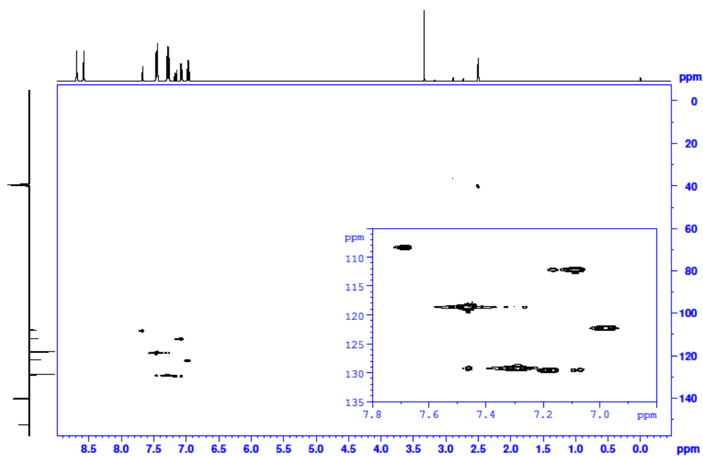
Slika P15. HSQC spektar spoja 5H_2 u DMSO- d_6 (400 MHz).
