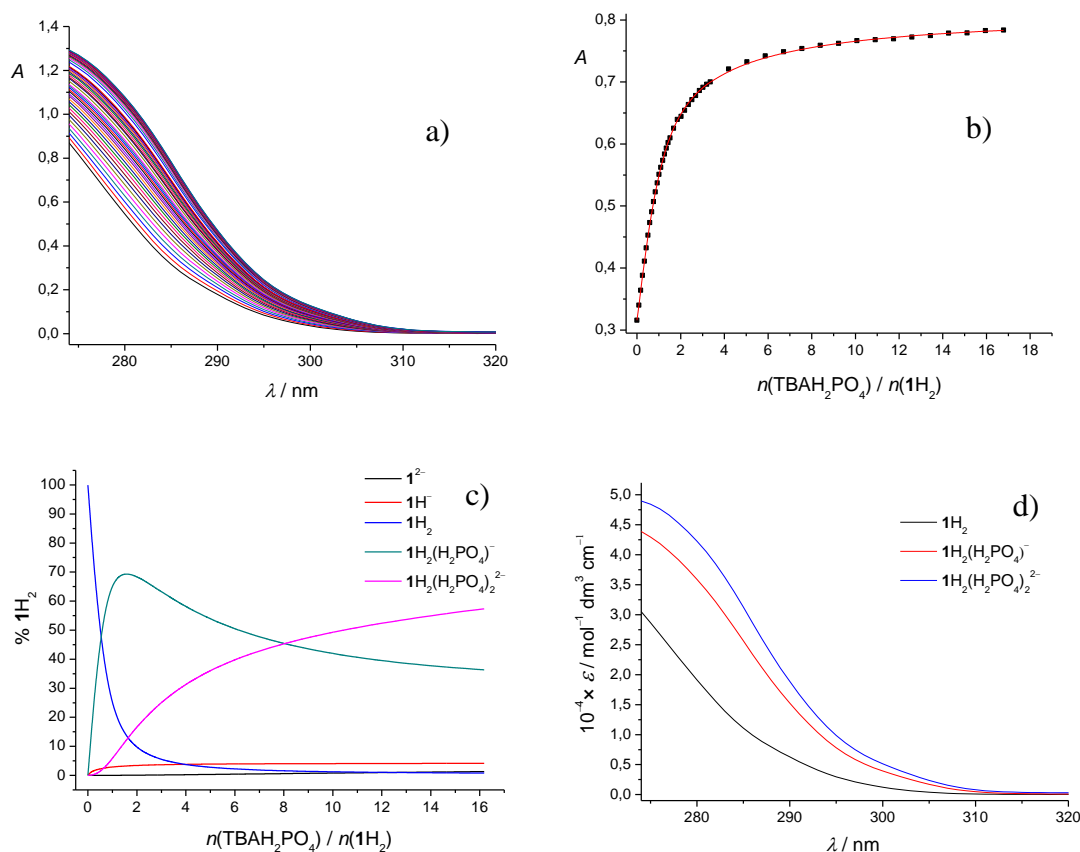
Slika 43. a) Spektrofotometrijska titracija 1H_2 ( c = 2,85 \times 10^{-5} \text{ mol dm}^{-3} ) s TBAH_2PO_4 ( c = 1,11 \times 10^{-3} \text{ mol dm}^{-3} ) u DMSO. Spektri su korigirani za razrjeđenje. l = 1 \text{ cm} , (25,0 \pm 0,1) \text{ }^\circ\text{C} . b) Ovisnost apsorbancije otopine 1H_2 pri 285 nm o množinskom omjeru n(TBAH_2PO_4) / n(1H_2) . ■ izmjerene vrijednosti, — izračunane vrijednosti. c) Distribucija pojedinih vrsta tijekom titracije otopine 1H_2 s TBAH_2PO_4 . d) Karakteristični UV spektri spoja 1H_2 i njegovih kompleksa s dihidrogenfosfatom.
