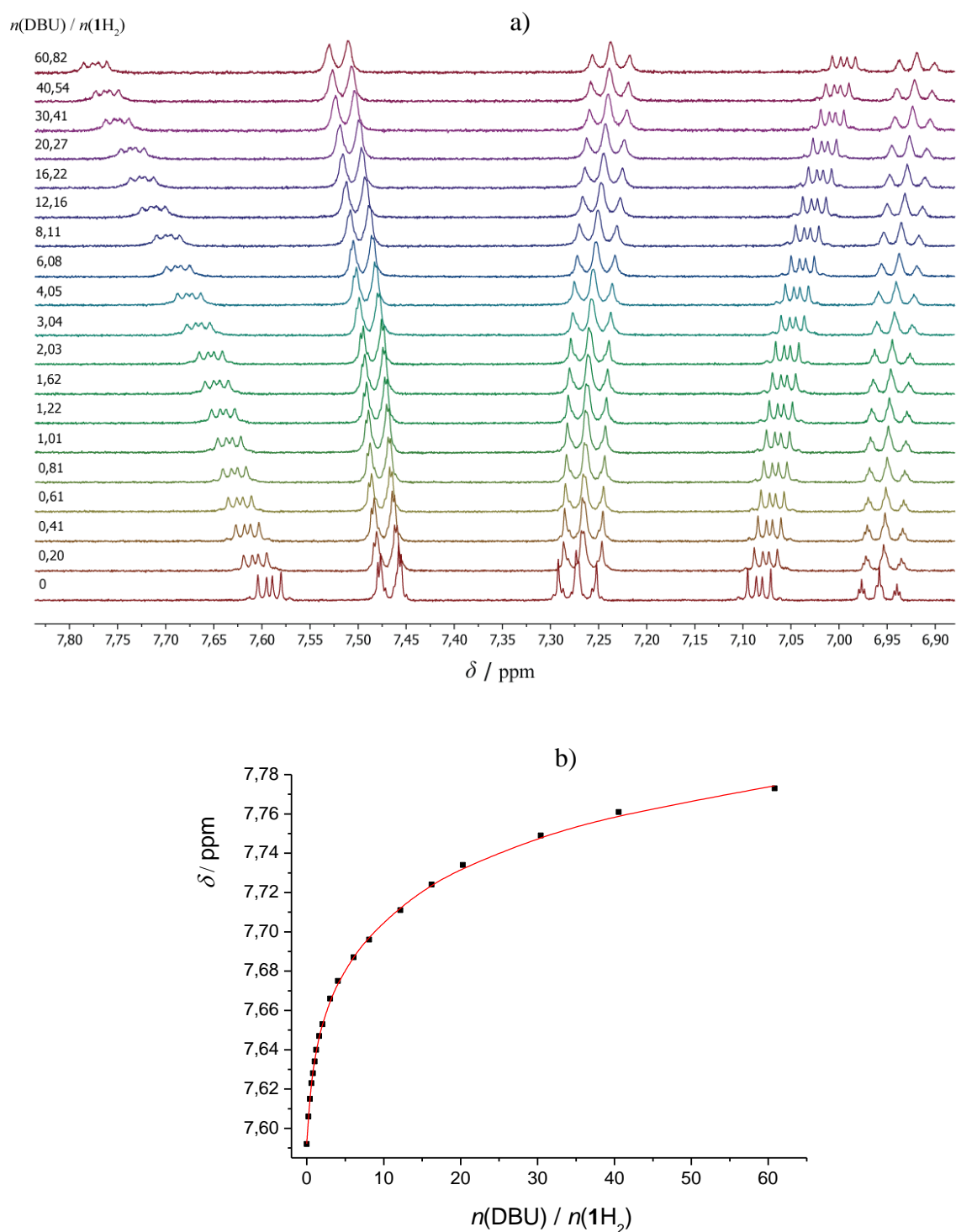
Slika 29. a) ^1\text{H} NMR titracija \mathbf{1H}_2 ( c = 5,94 \times 10^{-4} \text{ mol dm}^{-3} ) s DBU ( c = 6,32 \times 10^{-2} \text{ mol dm}^{-3} ) u DMSO- d_6 pri (25,0 \pm 0,1) \text{ }^\circ\text{C} . b) Ovisnost kemijskog pomaka \text{H}_b protona spoja \mathbf{1H}_2 tijekom ^1\text{H} NMR titracije s DBU o množinskom omjeru n(\text{DBU}) / n(\mathbf{1H}_2) . ■ izmjerene vrijednosti, — izračunane vrijednosti.
