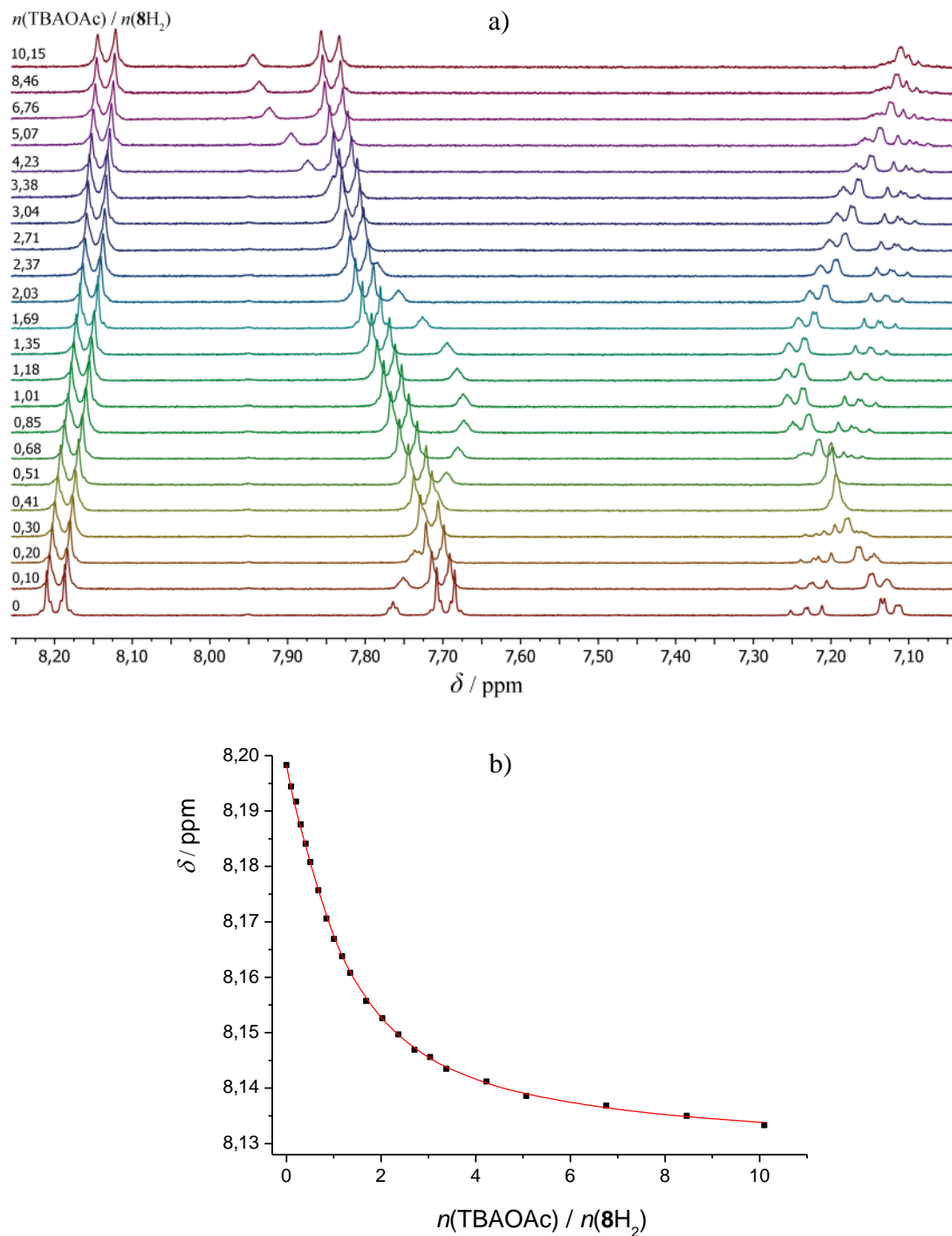
Slika 62. a) ^1\text{H} NMR titracija \mathbf{8H}_2 ( c = 5,86 \times 10^{-4} \text{ mol dm}^{-3} ) s TBAOAc ( c = 1,04 \times 10^{-2} \text{ mol dm}^{-3} ) u \text{DMSO-}d_6 pri (25,0 \pm 0,1) \text{ }^\circ\text{C} . b) Ovisnost kemijskog pomaka \text{H}_e protona tijekom ^1\text{H} NMR titracije s TBAOAc o množinskom omjeru n(\text{TBAOAc}) / n(\mathbf{8H}_2) . ■ izmjerene vrijednosti, — izračunane vrijednosti.
