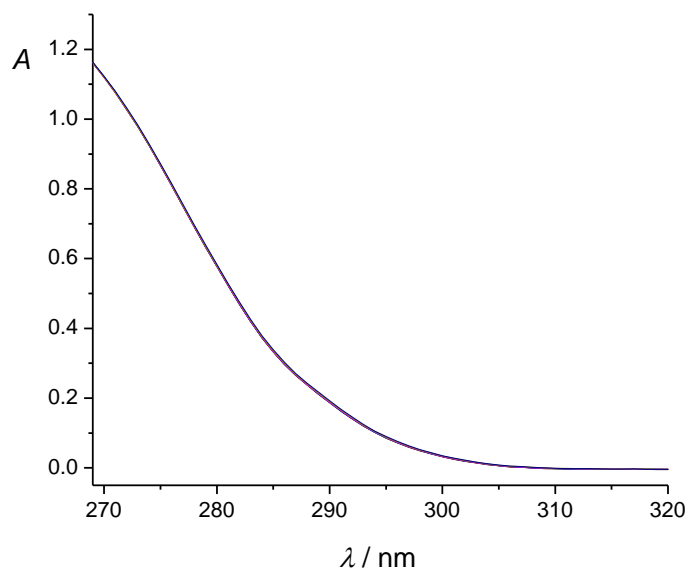
Slika P32. Spektrofotometrijska titracija 1H 2 ( c = 3,25 \times 10^{-5} \text{ mol dm}^{-3} ) s otopinom TBAClO 4 ( c = 7,03 \times 10^{-3} \text{ mol dm}^{-3} ) u DMSO. Spektri su korigirani za razrjeđenje. Množinski omjer n(\text{TBAClO}_4) / n(\mathbf{1H}_2) na kraju titracije iznosi 93. l = 1 \text{ cm} , (25,0 \pm 0,1) \text{ }^\circ\text{C} .
