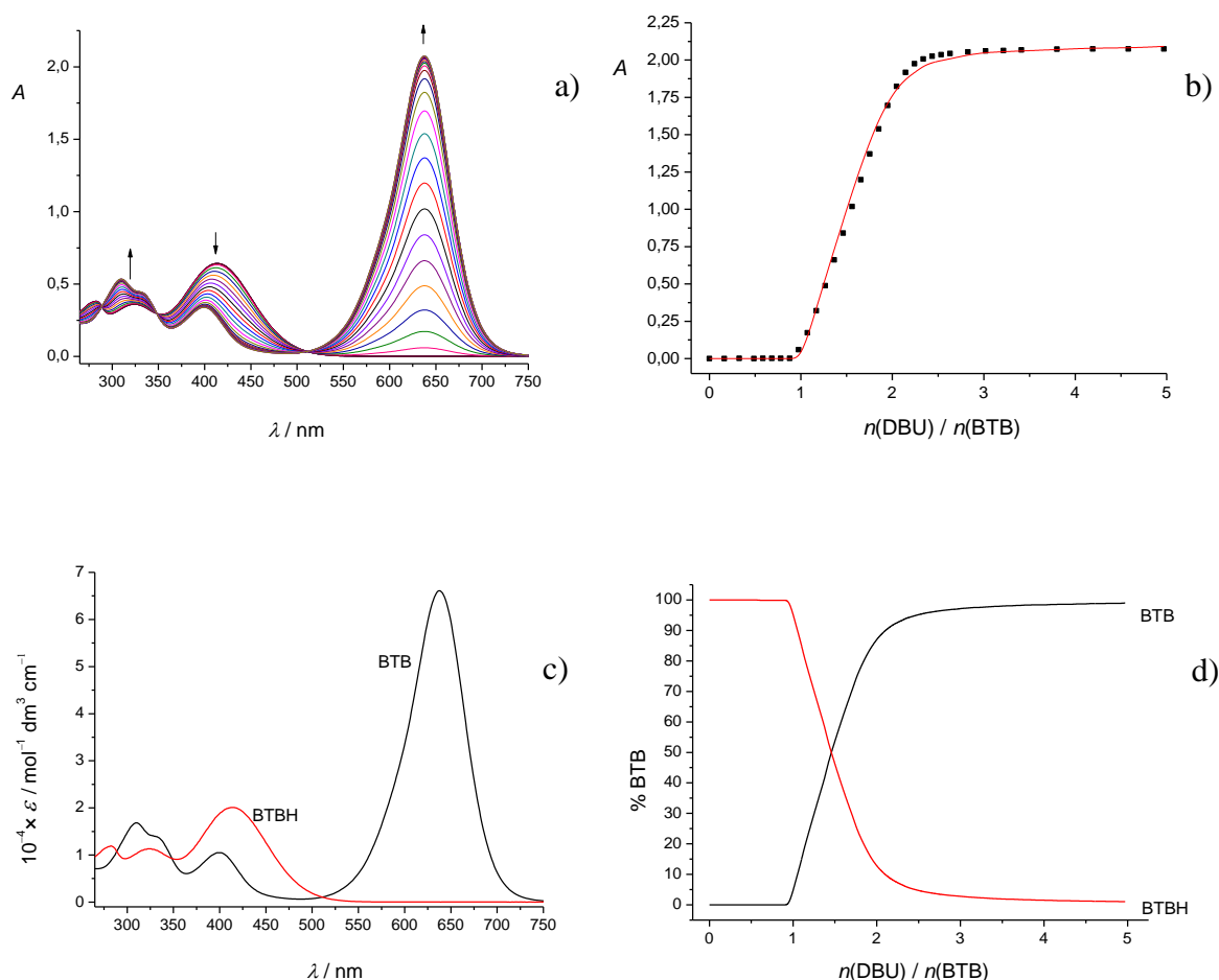
Slika 27. a) Spektrofotometrijska titracija bromtimol plavog ( c = 3,19 \times 10^{-5} \text{ mol dm}^{-3} ) s DBU ( c = 2,37 \times 10^{-3} \text{ mol dm}^{-3} ) u DMSO. Spektri su korigirani za razrjeđenje. l = 1 \text{ cm} , (25,0 \pm 0,1) \text{ }^\circ\text{C} . b) Ovisnost apsorbancije otopine bromtimol plavog pri 638 nm o množinskom omjeru n(\text{DBU}) / n(\text{BTB}) . ■ izmjerene vrijednosti, — izračunane vrijednosti. c) Karakteristični UV-Vis spektri protonirane i deprotonirane forme bromtimol plavog. d) Distribucija pojedinih vrsta tijekom titracije otopine bromtimol plavog s DBU.
