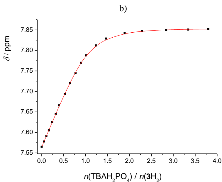
Slika 48. a) ^1\text{H} NMR titracija 3\text{H}_2 ( c = 6,10 \times 10^{-4} \text{ mol dm}^{-3} ) s \text{TBAH}_2\text{PO}_4 ( c = 8,78 \times 10^{-3} \text{ mol dm}^{-3} ) u \text{DMSO-}d_6 pri (25,0 \pm 0,1) \text{ }^\circ\text{C} . b) Ovisnost kemijskog pomaka \text{H}_b protona tijekom ^1\text{H} NMR titracije s \text{TBAH}_2\text{PO}_4 o množinskom omjeru n(\text{TBAH}_2\text{PO}_4) / n(3\text{H}_2) . ■ izmjerene vrijednosti, — izračunane vrijednosti.
