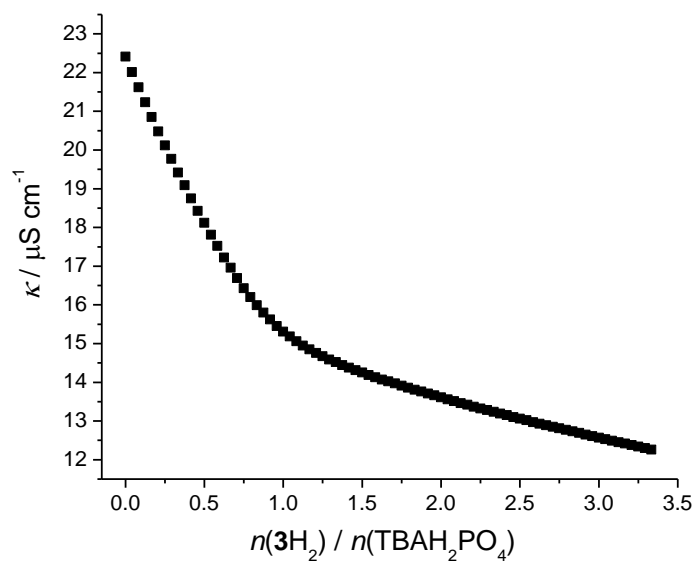
Slika P55. Ovisnost provodnosti otopine TBAH_2PO_4 o množinskom omjeru n(3H_2) / n(TBAH_2PO_4) tijekom konduktometrijske titracije TBAH_2PO_4 ( c = 6,65 \times 10^{-3} \text{ mol dm}^{-3} ) s 3H_2 ( c = 9,96 \times 10^{-4} \text{ mol dm}^{-3} ) u DMSO pri (25,0 \pm 0,1) ^\circ C .
