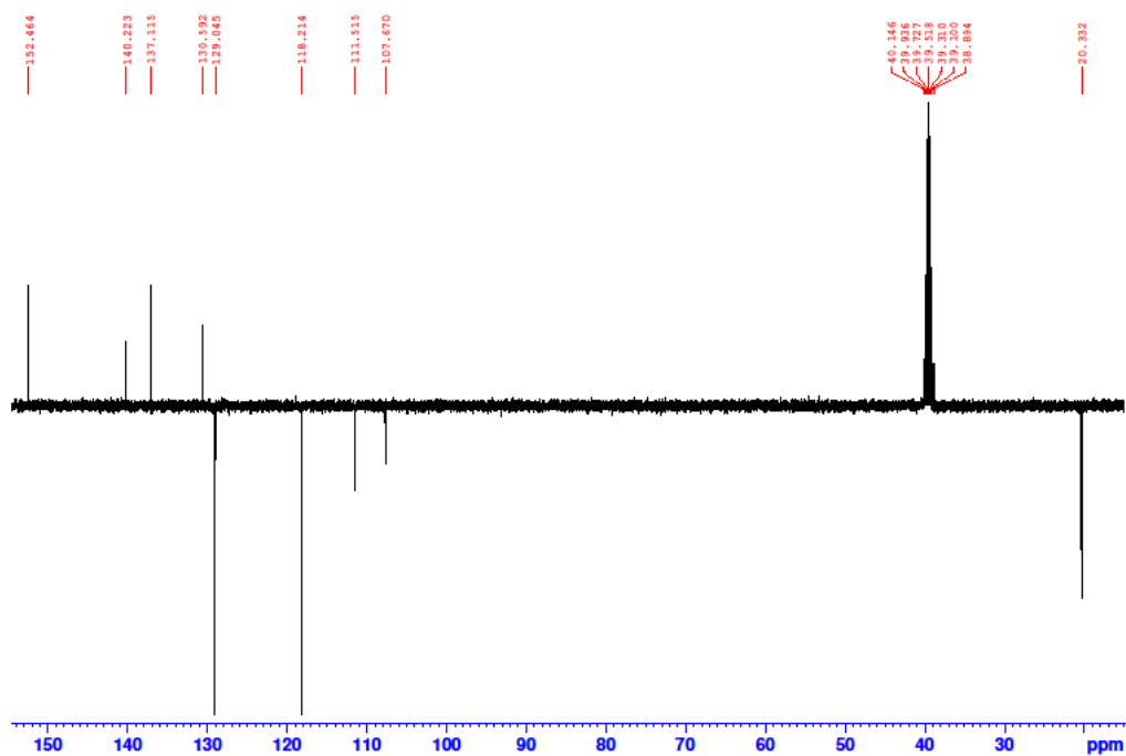
Slika P18. ^{13}\text{C} NMR spektar spoja 6\text{H}_2 u \text{DMSO-}d_6 (400 MHz).
