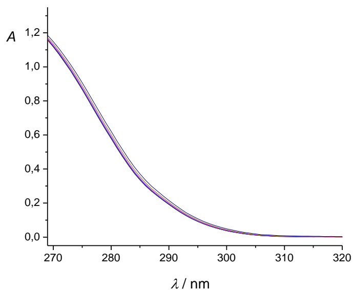
Slika P31. Spektrofotometrijska titracija 1H 2 ( c = 3,25 \times 10^{-5} \text{ mol dm}^{-3} ) s otopinom TEACl ( c = 7,80 \times 10^{-3} \text{ mol dm}^{-3} ) u DMSO. Spektri su korigirani za razrjeđenje. Množinski omjer n(\text{TEACl}) / n(\mathbf{1H}_2) na kraju titracije iznosi 103. l = 1 \text{ cm} , (25,0 \pm 0,1) \text{ }^\circ\text{C} .
