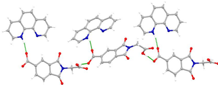
Slika 2.11. Motiv povezivanja ionâ u strukturi soli N -(karboksimetil)-7-karboksiftalimida i fenantrolina. Molekule kiseline povezane su u lanac O-H\cdots O vodikovim vezama, a fenantrolinijev kation vezan je na aromatske karboksilne skupine N-H\cdots O vodikovim vezama.
