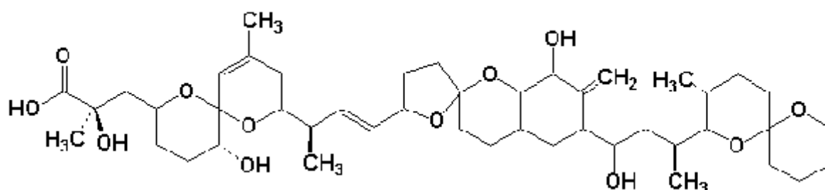
Slika 1. Strukturni prikaz molekule okadai ne kiseline
