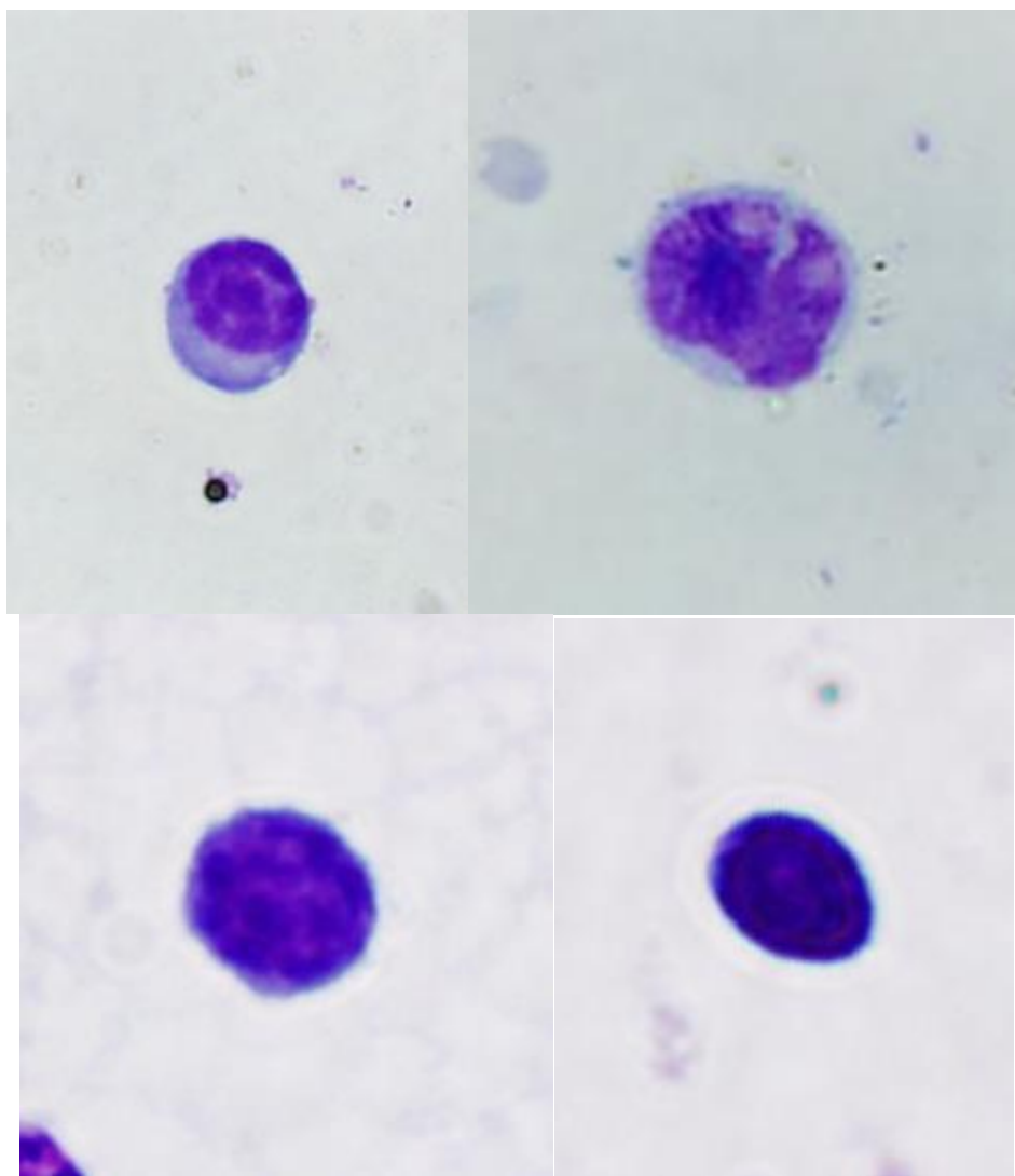
Slika 18. Prohemociti-MGG
