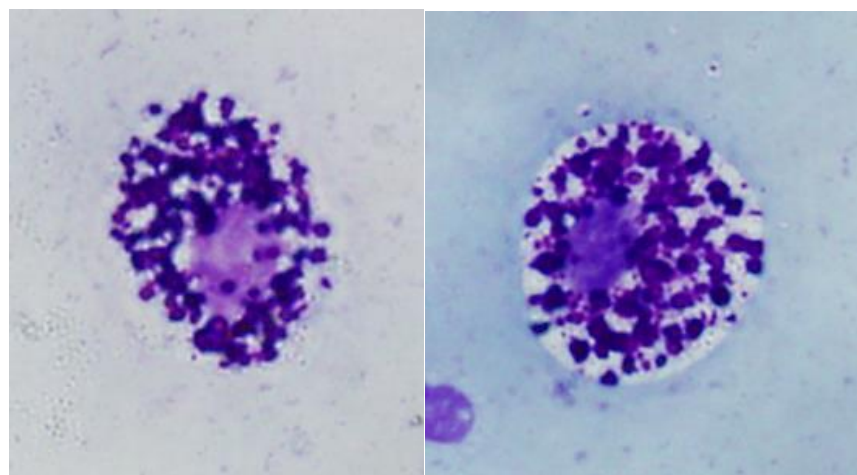
Slika 15. Granulociti-MGG
