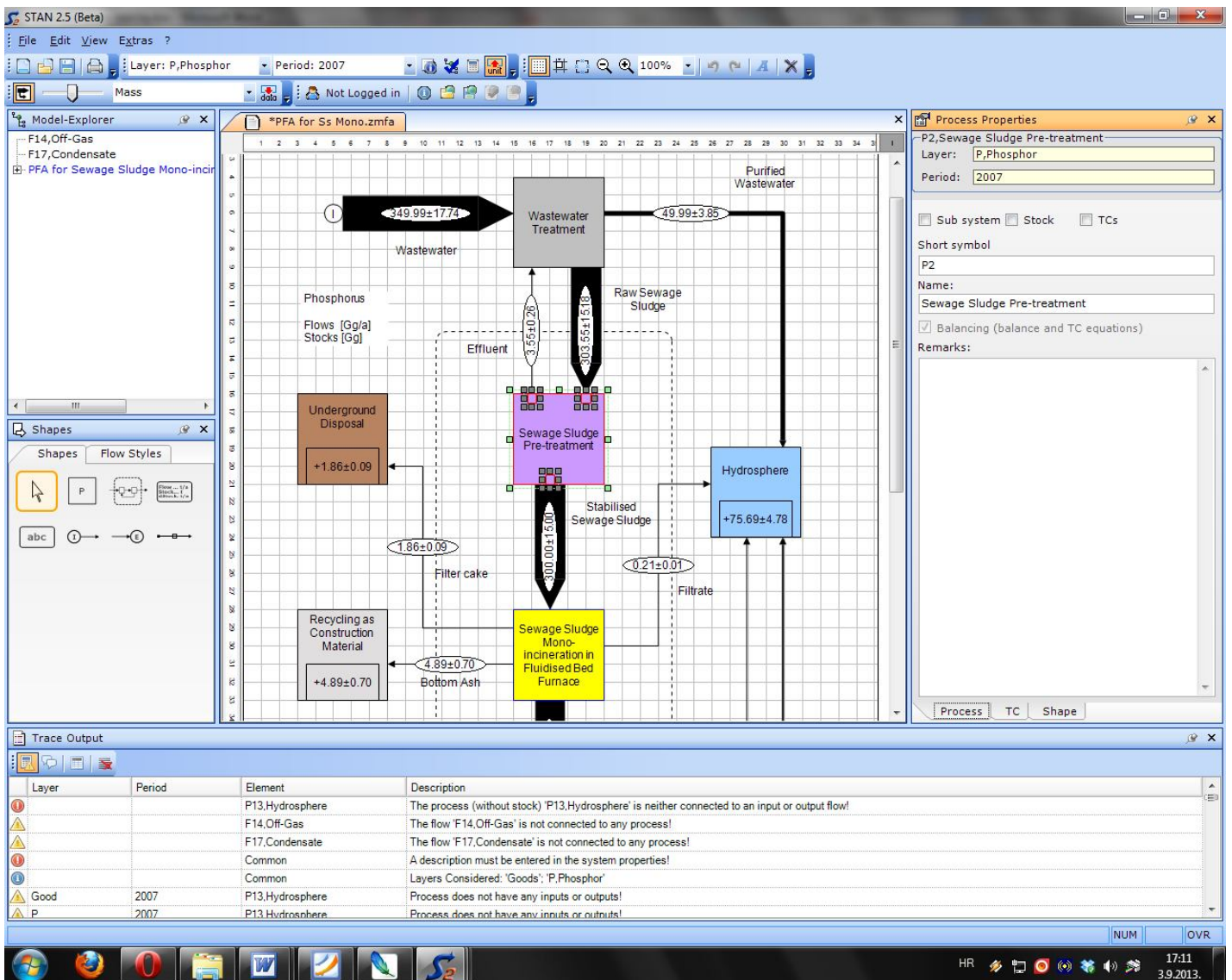
Slika 9: Grafičko sučelje STAN-sofvera nakon izračuna toka fosfora u sustavu koji prati fosfor u procesu spaljivanja aktivnog mulja.
