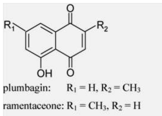
Slika 4. Kemijska struktura plumbagina i ramentaceona (preuzeto iz Babula i sur, 2006)
