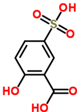
Slika 1. Strukturna formula 5-sulfosalicilne kiseline 15
