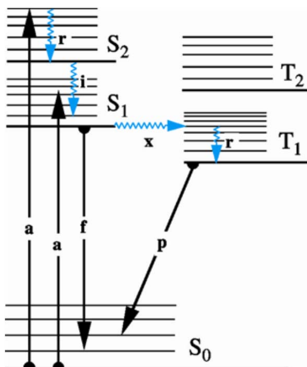
Slika M4. Dijagram Jablonskoga : radijativni prijelazi prikazani su ravnim strelicama, neradijativni vijugavim.(i - interna konverzija, r - vibracijska relaksacija, x – međusustavno križanje, a - apsorpcija, f - fluorescencija, p - fosforescencija) 25
