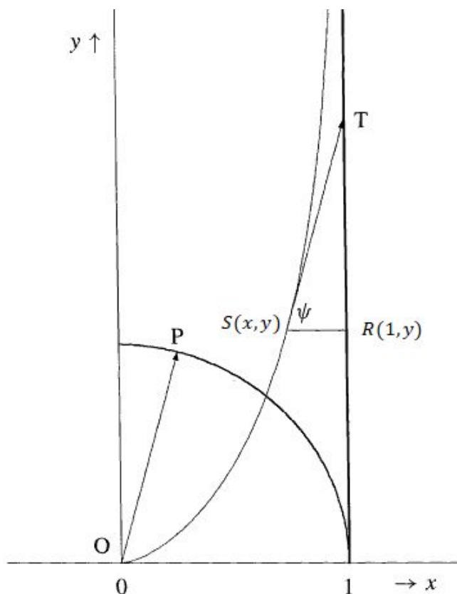
Slika 3.3: Traktrisa
