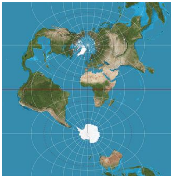
Slika 4.4: Transverzalni Mercator na sferi s obzirom na Grinički meridijan
