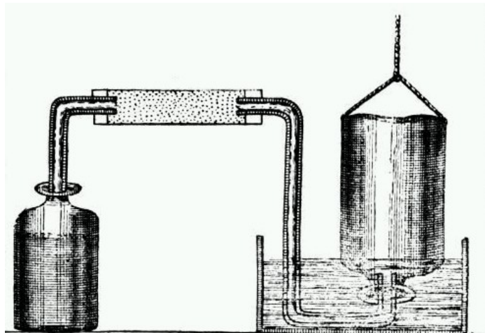
Slika 2.2: Skica Cavendishove aparature pomoću koje je dobio vodik. 5
