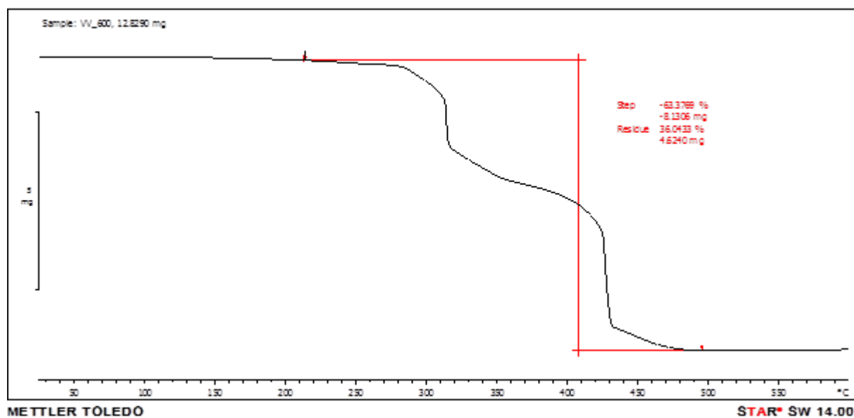
Slika D6. Termogravimetrijska analiza kompleksa [\text{MoO}_2(\text{VanNH})]_n do 600°C u struji \text{O}_2 , brzinom 5°C/min
