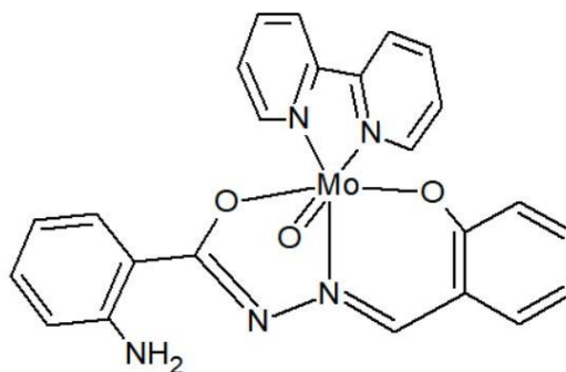
Slika 15. Pretpostavljena struktura kompleksa [\text{MoO}(\text{Sal-2-HBNH}_2)(\text{bipy})]
