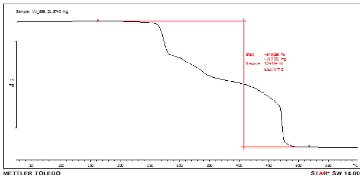
Slika D8. Termogravimetrijska analiza kompleksa [\text{MoO}_2(\text{H}_4\text{OMeSalNH})\text{Cl}]
