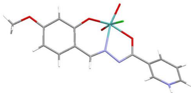
Slika 30. Molekulska struktura kompleksa [\text{MoO}_2(\text{H4OMeSalNH})\text{Cl}]
