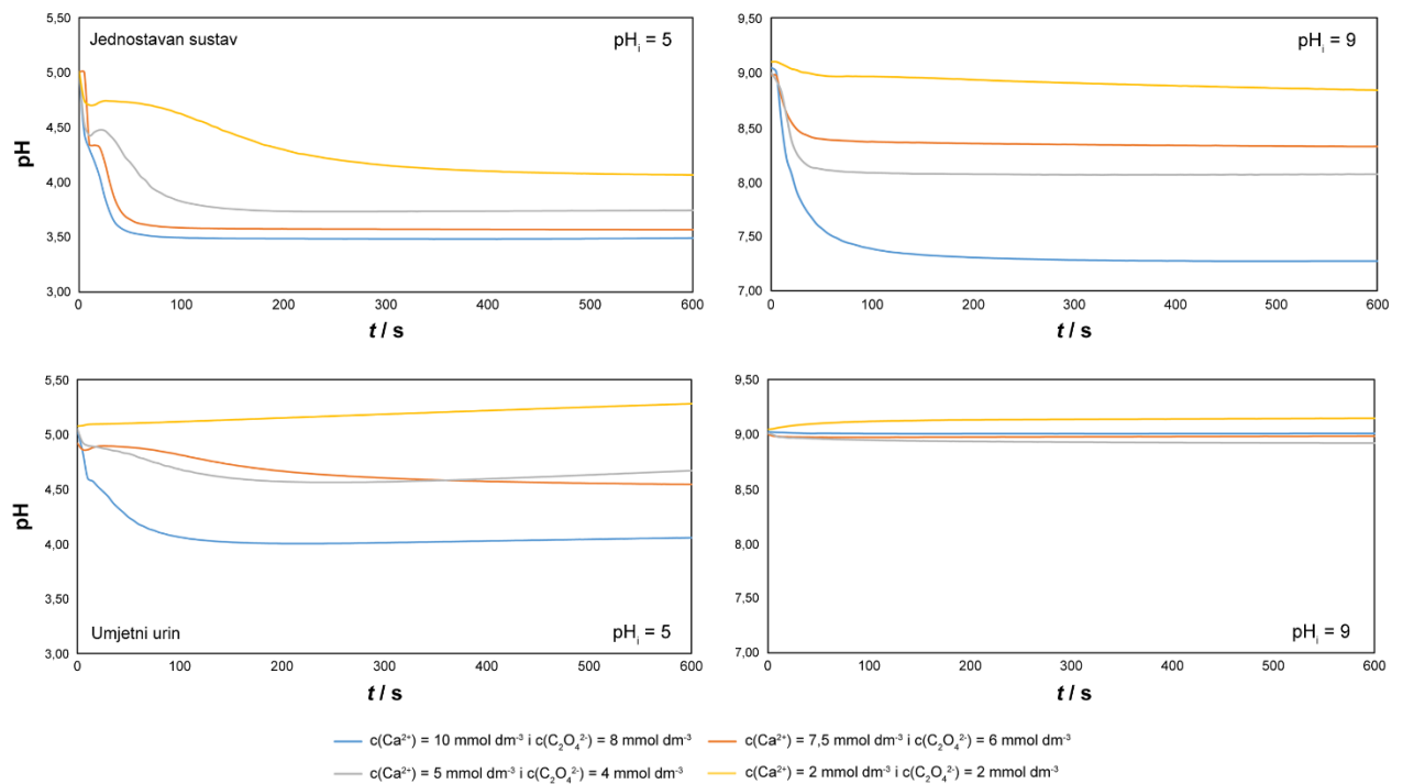
Slika 26. Ovisnost pH o vremenu spontanog taloženja kalcijeva oksalata pri različitim početnim koncentracijama reaktanata u jednostavnom sustavu i umjetnom urinu pri \text{pH}_i = 5 i \text{pH}_i = 9 .
