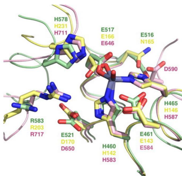
Slika 3. Preklopljene strukture mjesta za vezanje cinka kvašceve DPP III (zeleno), termolizina (žuto) i neprilizina (ružičasto). Slika je preuzeta iz rada Barala i suradnika. 14
