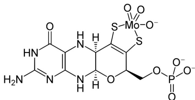
Slika 9. Molibdopterinski kofaktor 14 .
