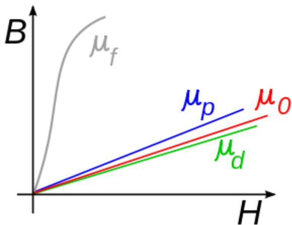
Slika 3. Ovisnost magnetske indukcije o magnetskom polju
