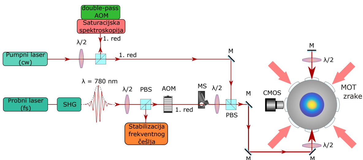
Slika 3.4: Shema eksperimentalnog postava dovođenja pumpnog i probnog lasera do oblaka hladnih atoma. Oznake: PBS - polarizacijski djelatelj zrake, M - zrcalo, \lambda/2 , \lambda/4 - polarizacijske pločice, AOM - akusto-optički modulator, SHG - generator drugog harmonika, MS - mehanički zatvarač, CMOS - kamera. Prilagođeno po uzoru na [22].
