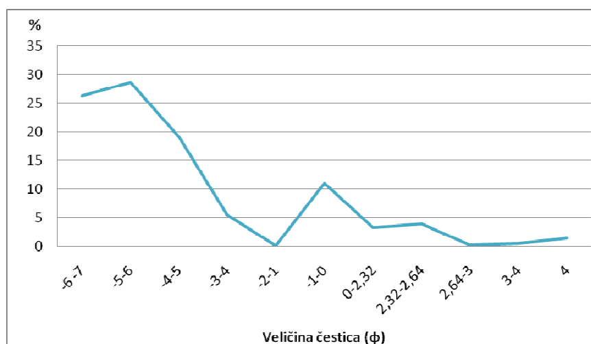
Slika 12. Krivulja učestalosti veličina čestica u uzorku Marasovići.
