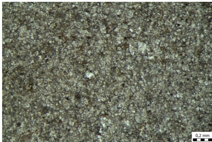
Slika 38. Ranodijagenetski dolomit.
