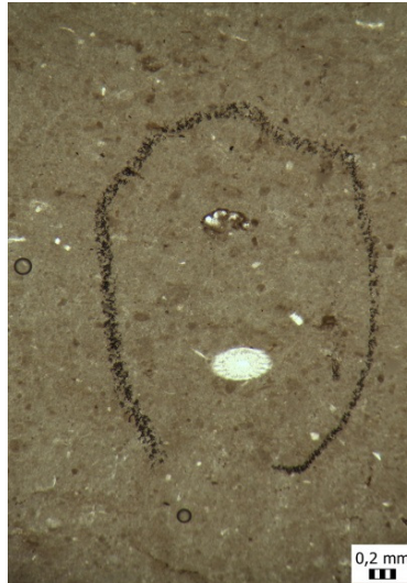
Slika 33. Fosiliferni mikrit.
