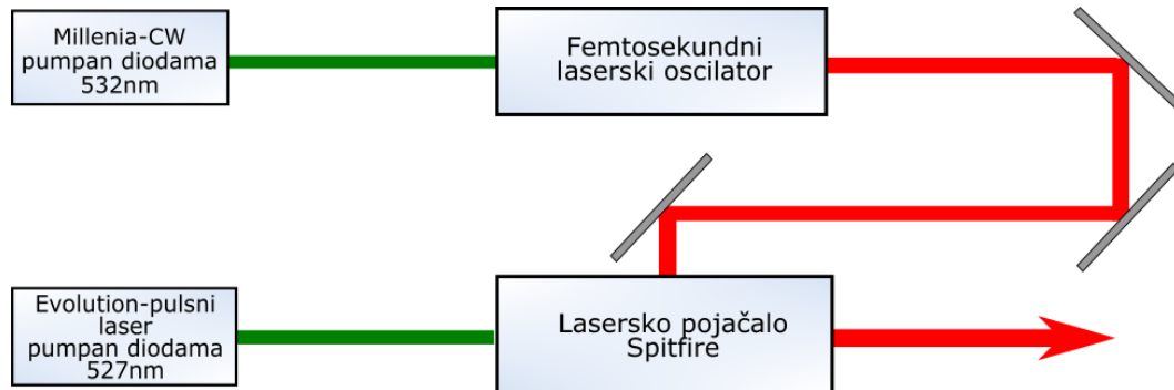
Slika 6.1: Shematski prikaz laserskog sustava.
