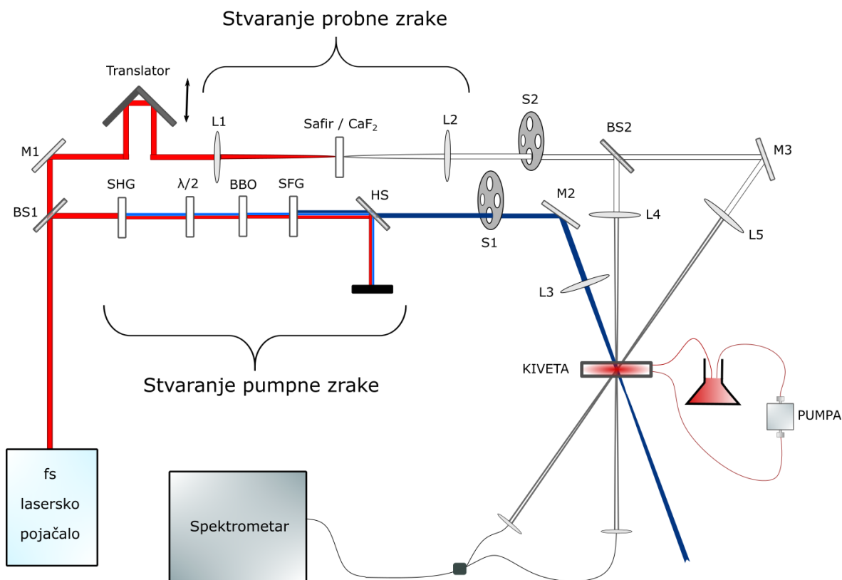
Slika 6.11: Postav za ultrabrznu tranzijentnu apsorpciju korišten u eksperimentu. Oznake: BS - djelitelji snopa, L - leće, M - zrcala, S - shutteri, HS - separatori harmonika.
