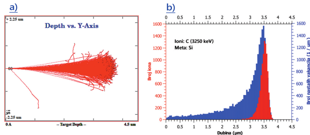
Slika 4.2: Rezultati TRIM simulacije upada 10000 iona ugljika, energije 3.25 MeV na Si metu. a) Prikaz putanje za 1000 iona kroz materijal. b) Prikaz raspodjele dosega upadnih iona, kao i raspodjele nastalih vakancija po mikrometru putanje o mjestu formacije (dubini)
