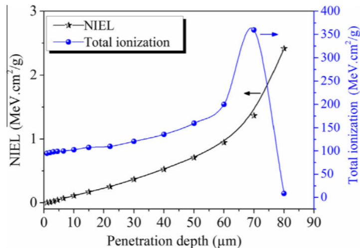
Slika 4.1: Prikaz izmjerenih vrijednosti ukupnog gubitka energije ionizacijom protona energije 2.55 MeV-a prilikom prolaska kroz silicijsku metu. Odsvojenom krivuljom je prikazana i NIEL komponenta. Izvor: [13]
