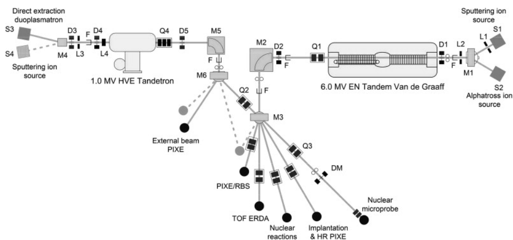
Slika 5.1: Shematski prikaz akceleratori sustava u sklopu LIIS laboratorija. Nuklearna mikroproba je na slici najdesnija od eksperimentalnih linija.
