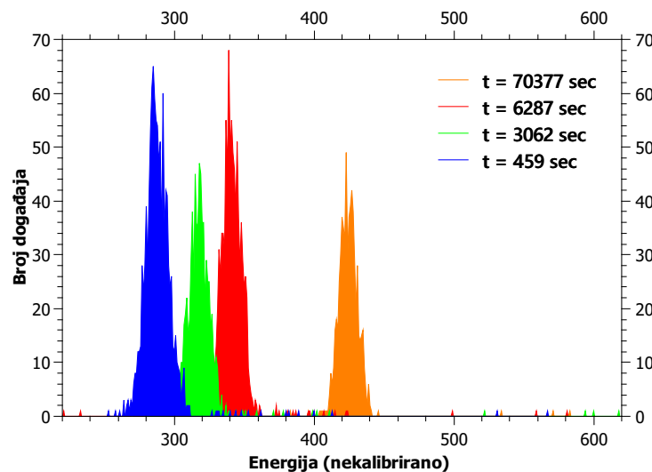
Slika 6.4: Zajednički prikaz energijskih spektara oštećenog dijela diode, ozračenog brzinom otklona snopa \eta_2 , u različitim vremenskim trenucima nakon prvotne radijacije. Nad maksimumima je provedena gausijanska prilagodba radi određivanja pozicije u energiji.
