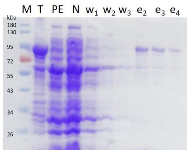
Slika 3.12. Poliakrilamidni gel (10%) nakon SDS-PAGE-a elucijskih uzoraka (e) nakon pročišćavanja na glutation-agaroznoj koloni. Slovom T je označen uzorak taloga nakon lize stanica, kraticom PE je označen supernatant nakon lize stanica, slovom N nevezana frakcija, te slovom w frakcije tijekom ispiranja nespecifično vezanih proteina. Slovo M označava marker molekulske masa Page Ruler® Prestained Protein Ladder .
