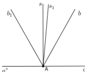
Slika 2.27: Dokaz Teorema 2.3.2 (3)
