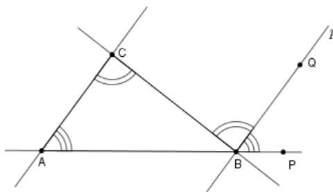
Slika 2.29: Dokaz Teorema 2.2.16
