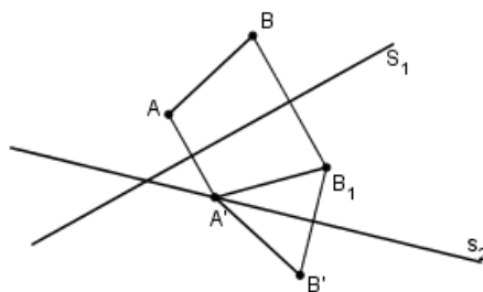
Slika 3.3: Dokaz Leme 3.2.9
