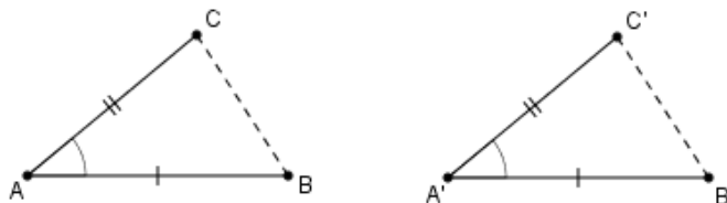
Slika 2.5: Lema 2.1.11
