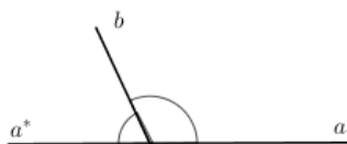
Slika 2.13: Sukut kuta \sphericalangle ab
