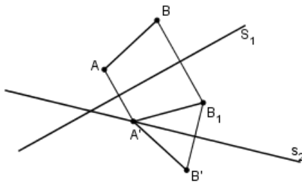
Slika 3.3: Dokaz Leme 3.2.9
