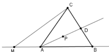
Slika 2.4: Teorem 2.1.10
