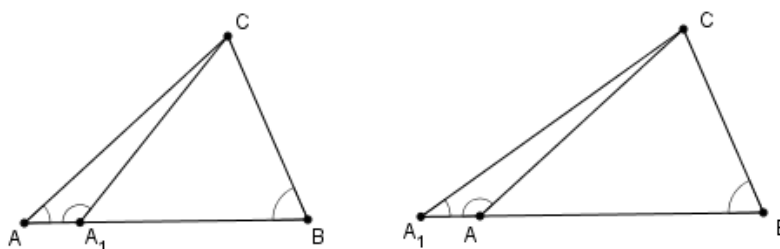
Slika 3.7: Dokaz Teorema 3.3.7
