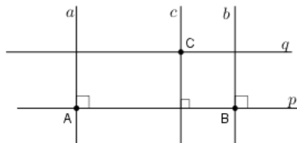
Slika 3.11: Dokaz Teorema 3.7.8
