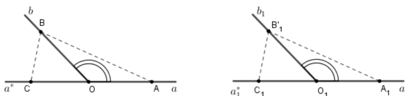
Slika 2.14: Dokaz Teorema 2.2.12
