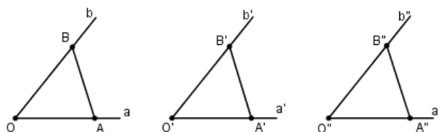
Slika 2.12: Dokaz Leme 2.1.17
