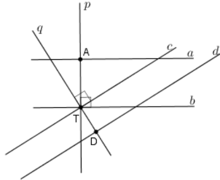
Slika 3.10: Dokaz Teorema 3.7.6
