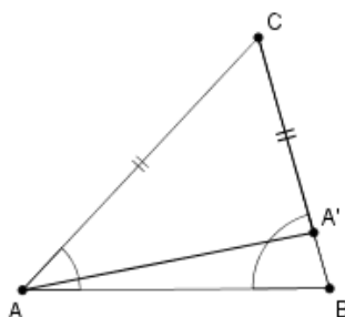
Slika 2.23: Dokaz Teorema 2.2.22 (2)
