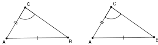
Slika 1.4: S-S-K^> teorem
