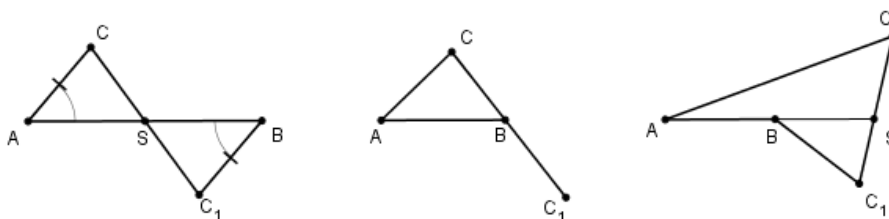
Slika 2.21: Dokaz Teorema 2.2.20
