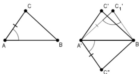
Slika 2.11: Dokaz Leme 2.1.16
