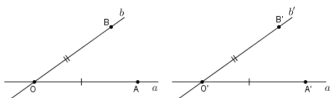
Slika 2.6: Dokaz Leme 2.1.12 (1)
