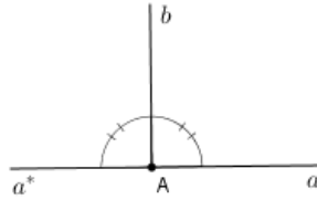
Slika 2.25: Dokaz Teorema 2.3.2 (1)
