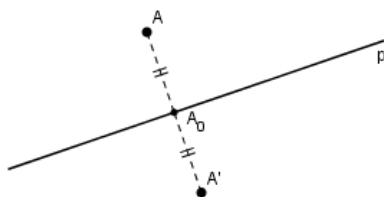
Slika 3.1: Dokaz Propozicije 3.1.2
