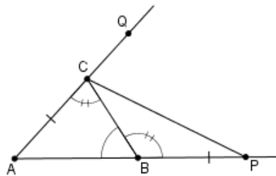
Slika 2.17: Dokaz Teorema 2.2.17 (2)
