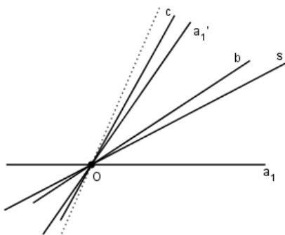
Slika 3.8: Dokaz Teorema 3.4.4
