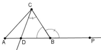
Slika 2.18: Dokaz Teorema 2.2.17 (3)
