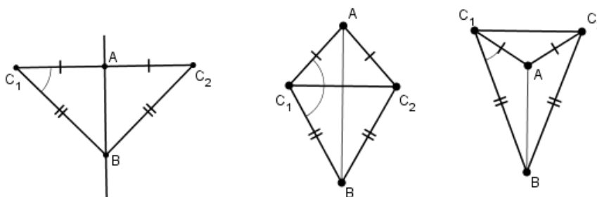
Slika 2.10: Dokaz Leme 2.1.15
