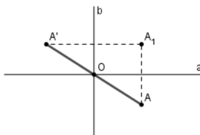
Slika 3.16: Centralna simetrija
