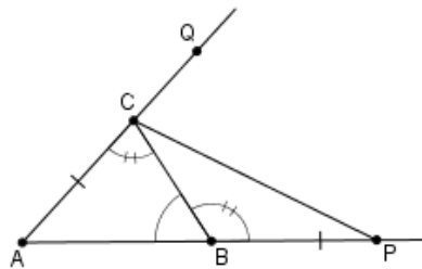
Slika 2.17: Dokaz Teorema 2.2.17 (2)
