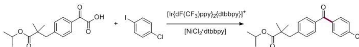
Shema 6. Reakcija pripreme fenofibrata fotokatalitičkim postupkom
