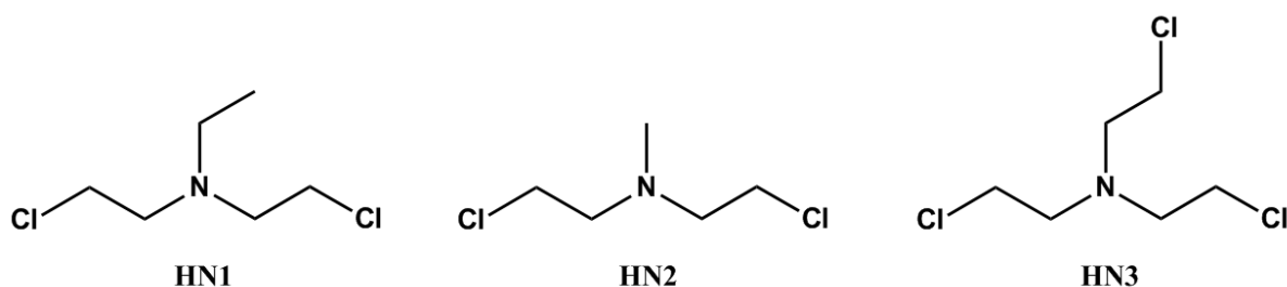
Slika 2. Strkturne formule odabranih analoga dušikovitih iperita (HN1 = N -etil- N -bis(2-kloretil)amin, HN2 = N -metil- N -bis(2-kloretil)amin, HN3 = N -tris(2-kloretil)amin)
