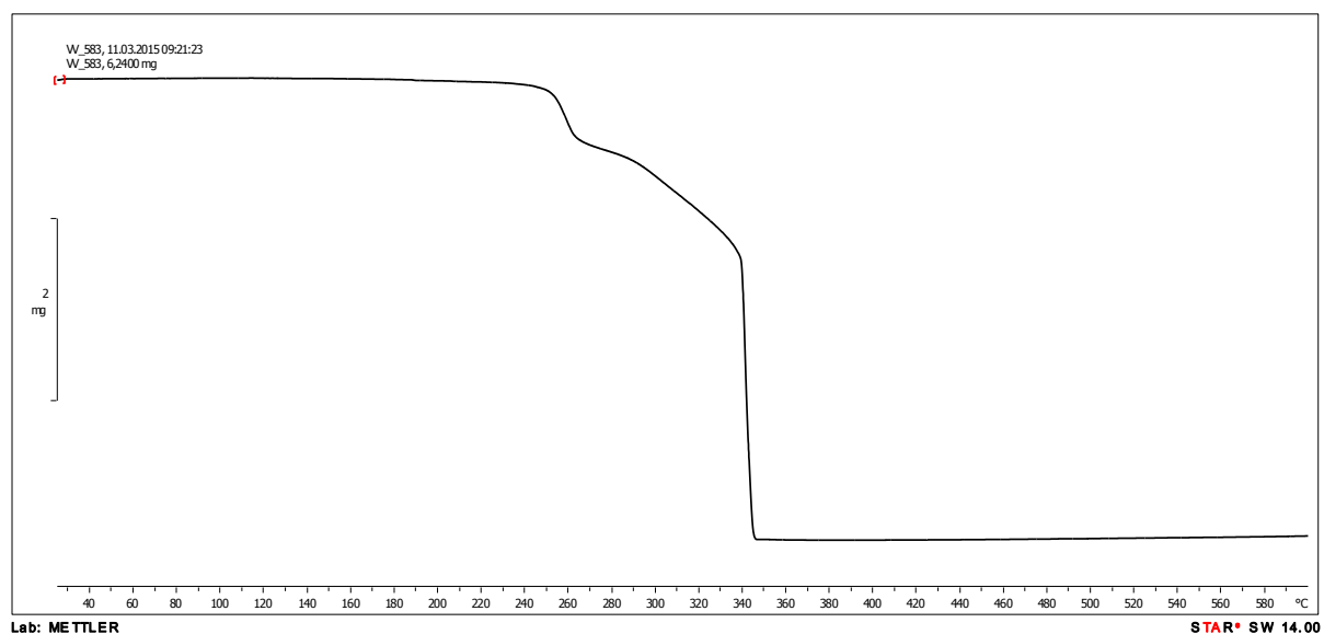
Slika 5.5. Termogravimetrijska krivulja kompleksa [\text{Ni}(\text{VanHBOH})(\text{py})] .
