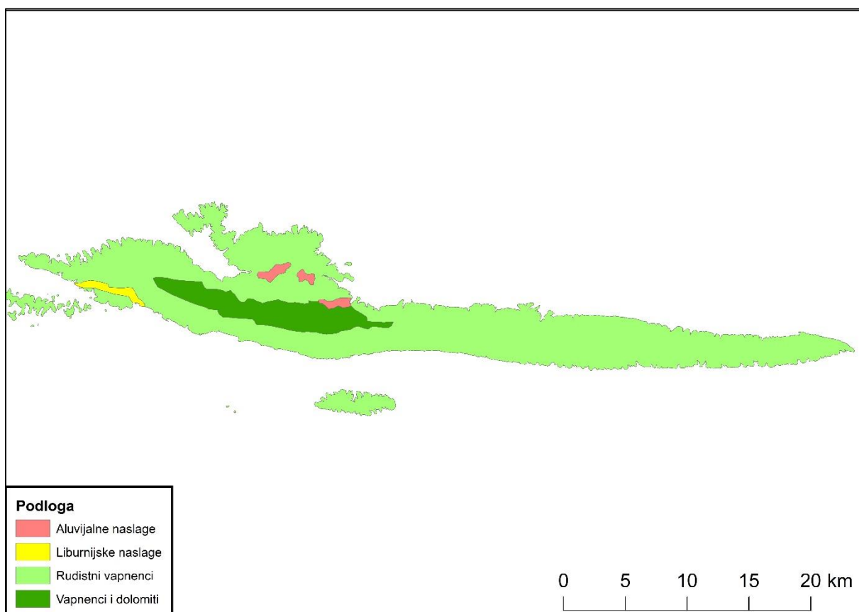
Sl. 2. Geološka osnova otoka Hvara
