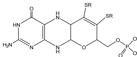
Slika 1. Struktura molibdopterina
