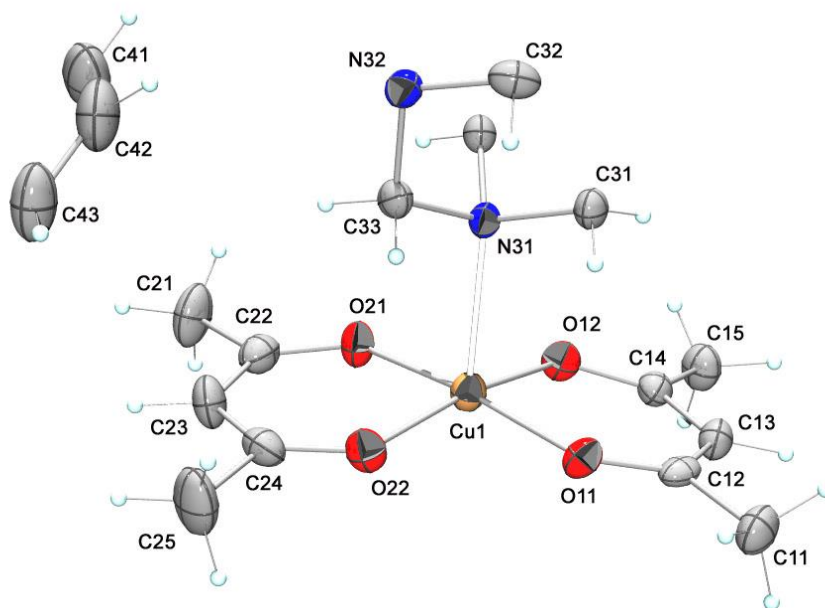
Slika 1. Crtež asimetrične jedinice kristala [\text{Cu}(\text{acac})_2](\text{hmta}) u kojem je prikazana i shema označavanja atoma. Radi preglednosti crteža prikazana je samo asimetrična jedinka, a ne cijeli molekularni kompleks. Vibracijski elipsoidi nevodikovih atoma odgovaraju 30 % vjerojatnosti elektronske gustoće, a vodikovi atomi prikazani su kao kuglice proizvoljnog radijusa. Crtež je načinjen programima ORTEP-3 i POV-Ray . 18,21
