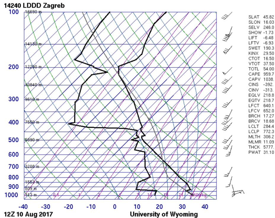
Slika 52. "Skew-T log-P" dijagram radiosondaže 10. kolovoza 2017. u 12 UTC. Izvor: internetske stranice Sveučilišta u Wyomingu, http://weather.uwyo.edu/upperair/sounding.html
