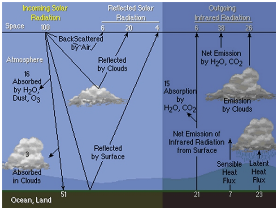
Slika 3.2: Komponente reflektiranog i apsorbiranog zračenja Sunca, Zemlje i atmosfere. ( https://www.met.ed.ucar.edu/asm1/asm1/media/graphics/graphic2.jpg )
