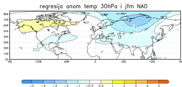
Slika 3.26 Regresijski koeficijent [°C/hPa] dobiven linearnom regresijom temperature na izobornoj plohi 30 hPa i NAO indeksa za JFM sezonu (podaci: NCEP-NCAR reanaliza za razdoblje 1948.-2015.). Izvor: NOAA/ESRL Physical Sciences Division; www.esrl.noaa.gov/psd/ .
