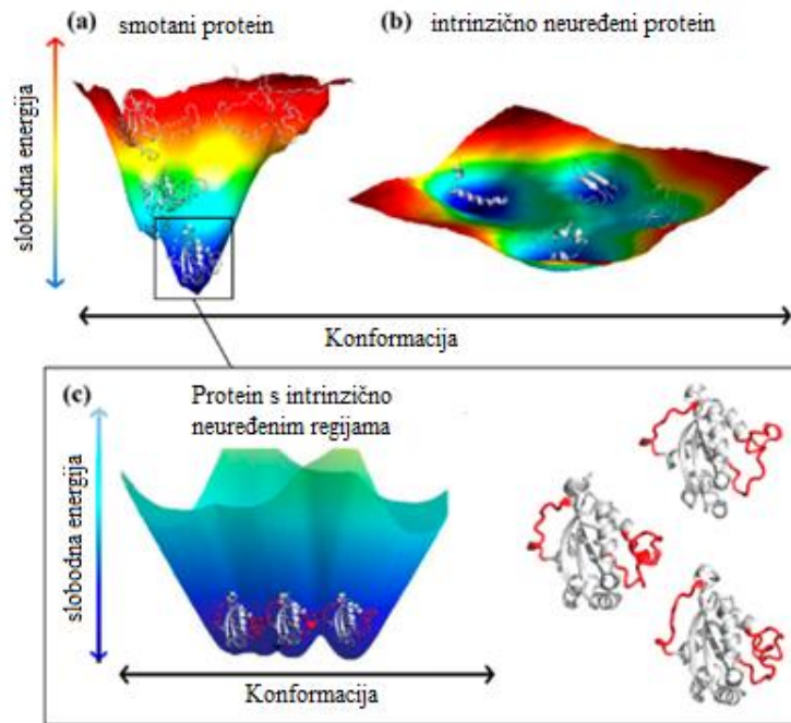
Slika 6. Shematski prikaz energetskega dijagrama smatanja za a) uređeni protein i b) INP, te c) uvećani prikaz dna energetskega dijagrama za protein s uređenim domenama povezanimi neuređenim linkerima. (Preuzeto i prilagođeno iz Uverski i sur. 2016.).
