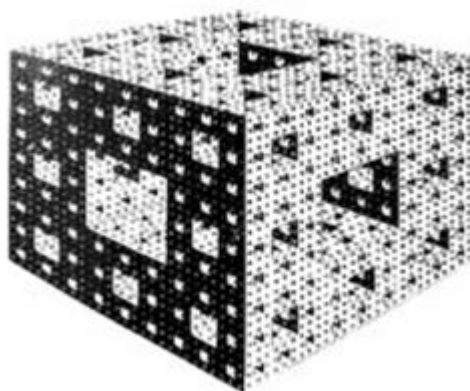
Slika 2.7: Mengerova spužva
