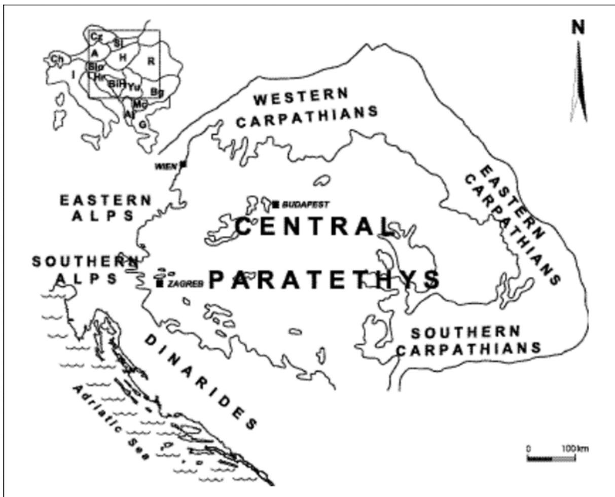
Slika 2. Prostiranje centralnog Paratethysa u kasnom badenu (preuzeto iz Pavelić 2002)
